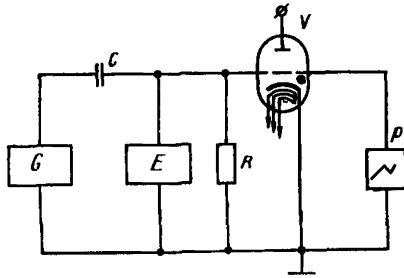
C — переходной конденсатор, E — фильтр, G — источник импульсного напряжения P — осциллограф, R — резистор угетки, V — ис- пытываемый тиратрон
