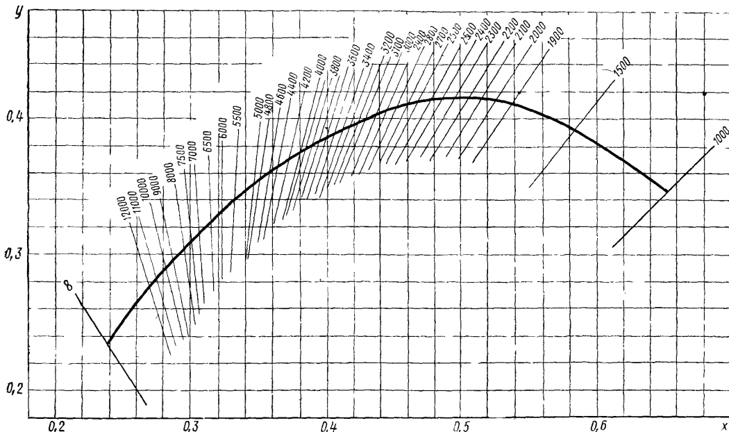
ГРАФИК ДЛЯ ОПРЕДЕЛЕНИЯ ЦВЕТОВОЙ ТЕМПЕРАТУРЫ ЭКРАНОВ КИНЕСКОПОВ ПО КООРДИНАТАМ ЦВЕТНОСТИ ИХ СВЕЧЕНИЯ
