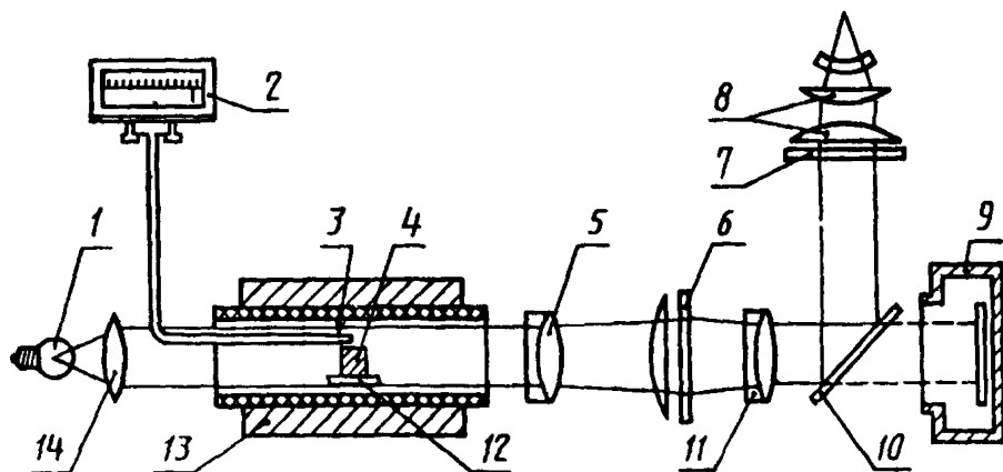
1 — осветителя, 2 — милливольтметр, 3 — термopара, 4 — образец из золы, 5 — координатная сетка, 7 — матовое стекло, 8 — линза, 9 — фотографическая камера, 10 — зеркало, 11 — окуляр, 12 — подставка, 13 — электропечь, 14 — конденсор
