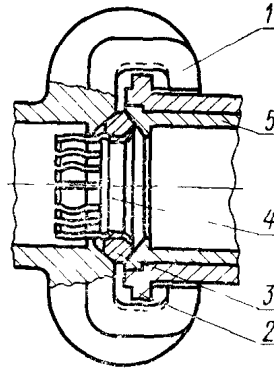
1, 2—гайки; 3—кольцо; 4— втулка; 5—штуцер
