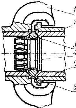
1, 2—гайки; 3—кольцо; 4—втулка, 5, 6—штуцер
