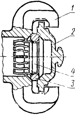
1, 2—гайки; 3—кольцо; 4—втулка.
