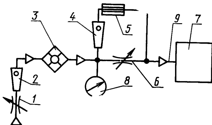
1—дроссель; 2—ротаметр 1; 3—испаритель анестетиков; 4—ротаметр 2; 5—устройство для измерения концентрации паров наркотизирующих веществ; 6—дроссель; 7—вытяжной шкаф; 8—манометр; 9—газоотводящий шланг.
