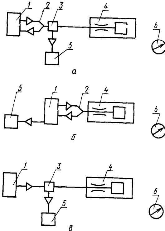
1—аппарат ИВЛ, 2—тройник пациента, 3—неревверсивный клапан, 4—модель легких, 5—спирометр, 6—секундомер
