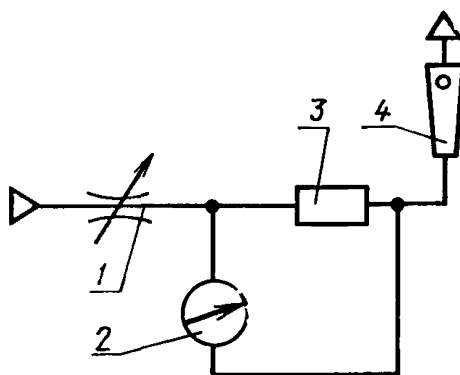
1—дроссель; 2—манометр; 3—аппарат; 4—ротаметр.
