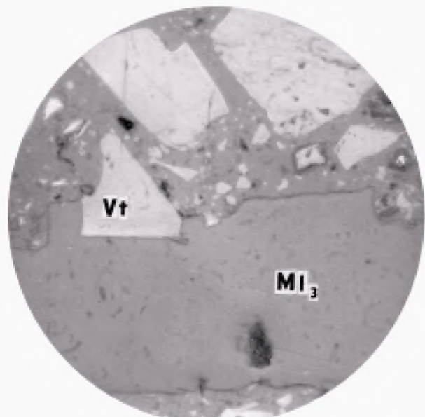
Сросток микролитотипа 1-й группы ( V ) + + кальцит ( MI_3 )
