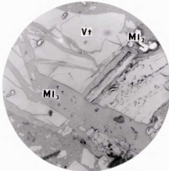
Сросток микролитотипа 1-й группы ( V_t ) + пирит ( MI_2 ) + кальцит ( MI_3 )
