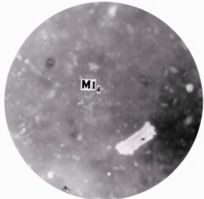
Известняк (M 4 ) (увеличение 200)
