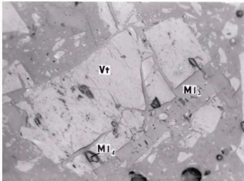
Сросток микролитотипа 1-й группы ( V_t ) + сидерит ( MI_3 ) + кварц ( MI_4 )
