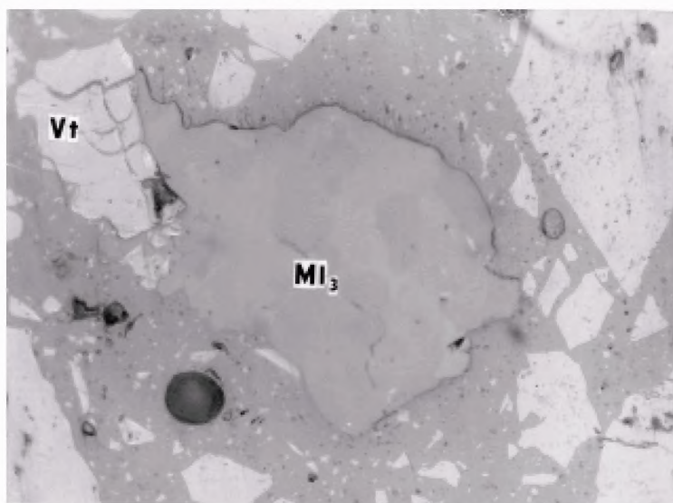
Сросток микролитотипа 1-й группы ( V_t ) + сидерит ( M_3 )
