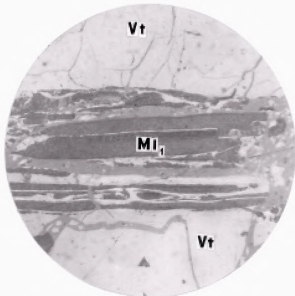
Сросток микролитотипа 1-й группы ( V ) + + каолинит ( MI_1 ) Черт. 7
