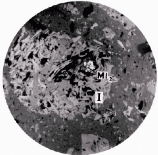
Сросток микролитотипа 3-й группы ( F ) + + пирит ( MI_2 )
