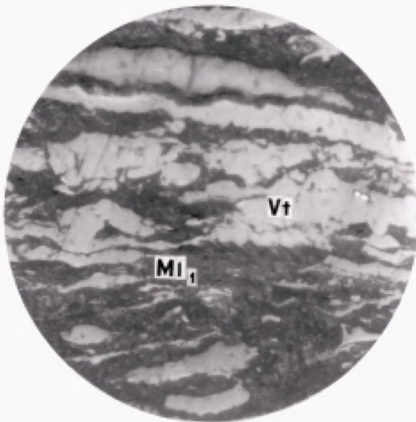
Сросток микролитотипа 1-й группы ( V ) + + аргиллит ( MI_1 )
