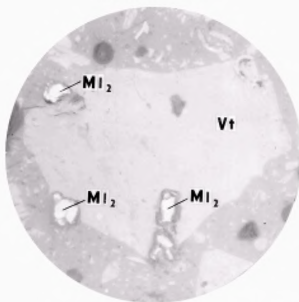
Сросток микролитотипа 1-й группы ( V ) + + пирит ( MI_2 ) Черт. 8
