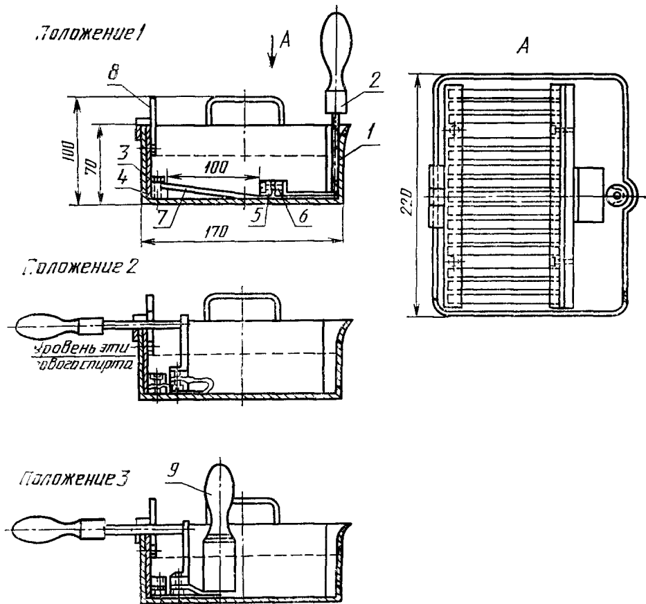
1—ванна, 2—ручка, 3—зажим 1, 4—брусок, 5—зажим 2, 6—брусок, 7—образцы, 8—защелка; 9—пестик
