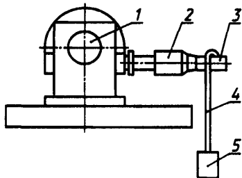
1 — привод; 2 — подвижный зажим; 3 — стержень; 4 — образец провода; 5 — нагрузка
