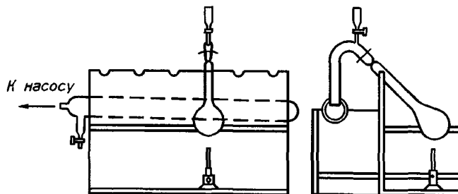
Рисунок 2 — Аппарат для мокрого окисления пробы
