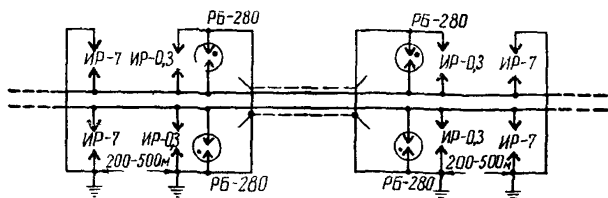
Рис.6. Защита разрядниками кабельных вставок (для кабелей с металлической оболочкой)
