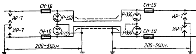
Рис.20. Защита разрядниками кабельной вставки на воздушной линии местной связи (для кабелей с металлической оболочкой)
