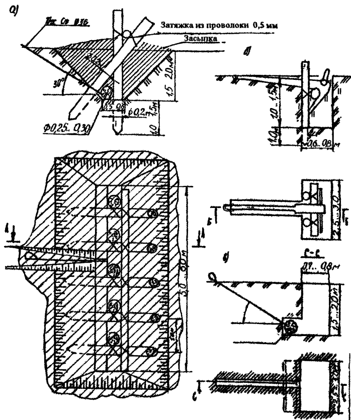
Рис. П. 2.3. Устройство якоря - "мертвяка"
