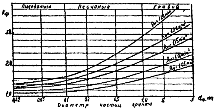
Рис. 17. График определения коэффициента, учитывающего увеличение потерь напора в трубопроводе от грунта.
