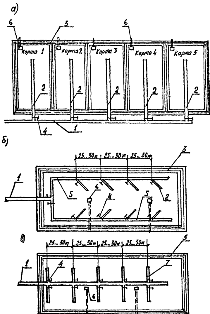
Рис. П. 7.4. Схема намыва:
