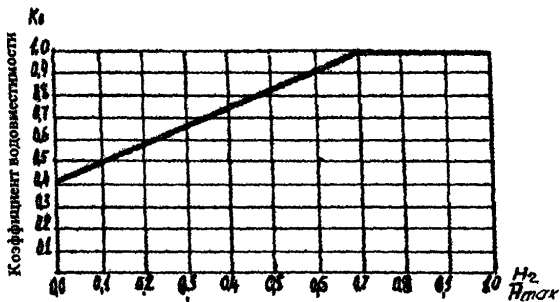
Рис.22. Предельные перемещения земснаряда вперед, коэффициент водовместимости черпака а - предельное перемещение земснаряда, б. - коэффициент водовместимости черпака.
