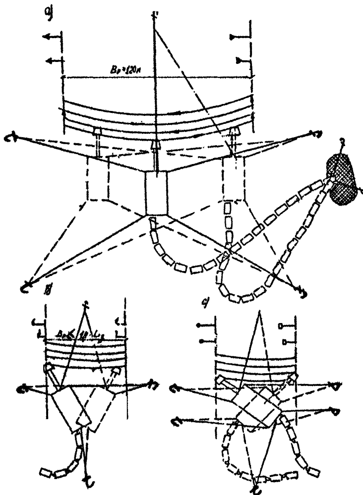
Рис.16. Рабочие перемещения на прорези авантово-папильонажного землесоса
