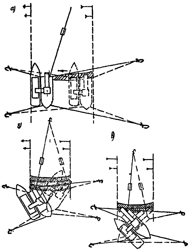
Рис.19. Способы перемещения многочерпакового земснаряда на прозеи : а - параллельный, б - веерный, в - крестовый.
