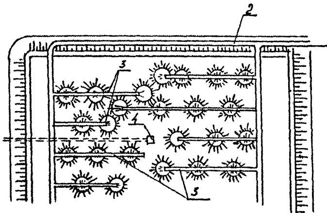
Рис. II. 7.5. Мозаичный способ намыва
