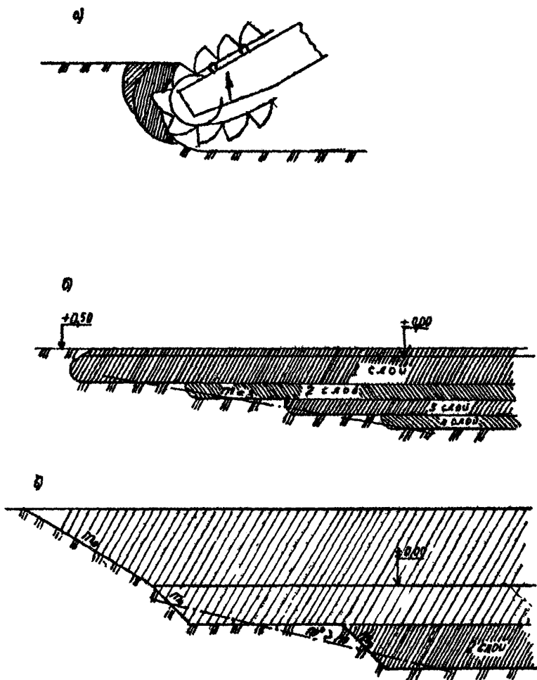
Рис.21. Схема разработки на мелководье и в сухом берегу
