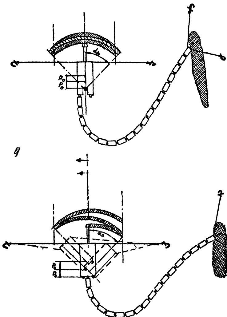
Рис.15. Схема перемещения на прорези свайно-папильонажных землесосов а) - Земснаряд с напорным свайным ходом; б) - Земснаряд с шагающим свайным ходом; P_0 - перемещение земснаряда вперед, \alpha_n - угол разворота земснаряда при выходе на бровку
