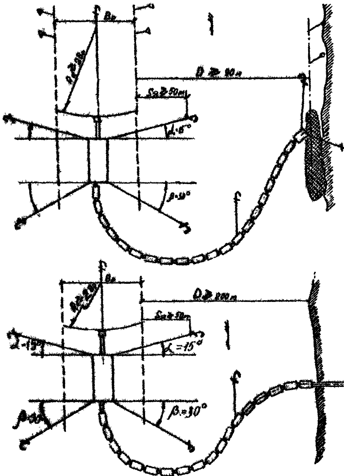
Рис. 1. Схема установки на участке работ цепильонажного землесоса B_p - рабочая ширина прорези, D - удаленность отвала грунта от бровки, R_x - радиус качания земснаряда на аванте, S_d - дальность завозки рабочего якоря от бровки, \alpha - угол опережения рабочего троса, \beta - угол отставания рабочего троса
