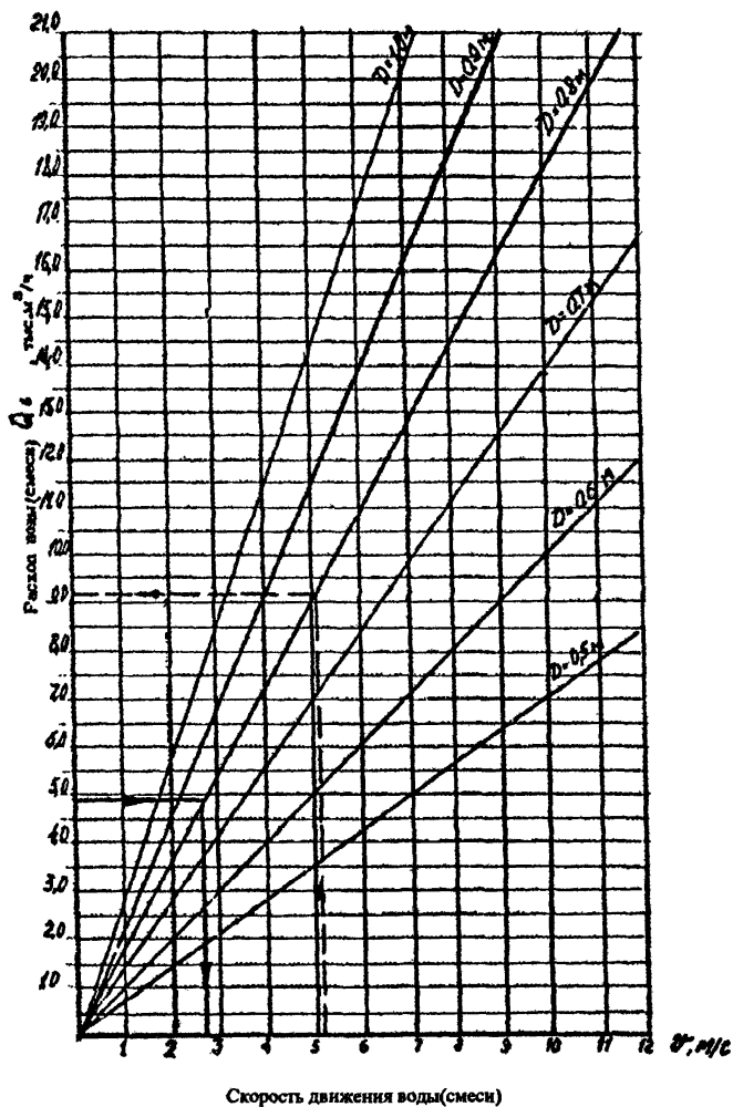
Скорость движения воды(смеси) Рис. П. 5.1. График для определения расхода и скорости смеси в грунтопроводе
