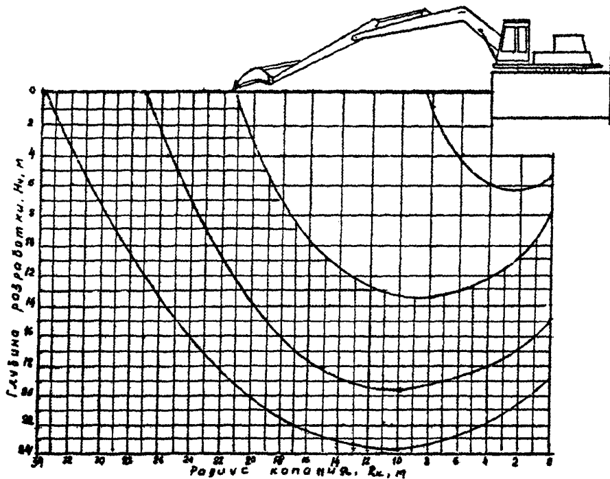
Рис.27. Радіус копанія штангового земснаряда «обратная лопата»
