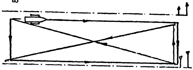
Рис.11. Подрезка бровок путем создания вдоль бровок траншей 1- наносы, 2- траншеи вдоль бровок а)
