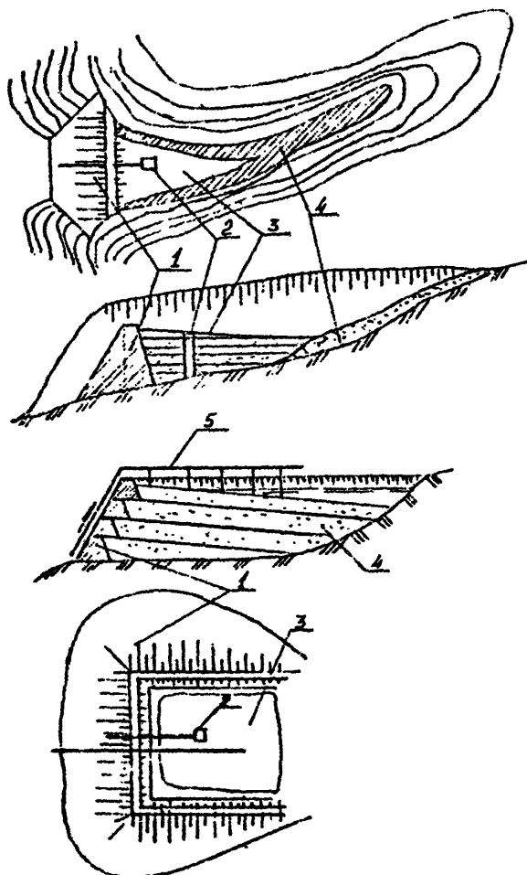
Рис. П. 7.9. Укладка грунта в гидроотвал. а- в овраге, б- на береговом откосе, 1- обвалование, 2- сбросный колодец, 3- прудок, 4- насыпный грунт, 5- грунтпровод.
