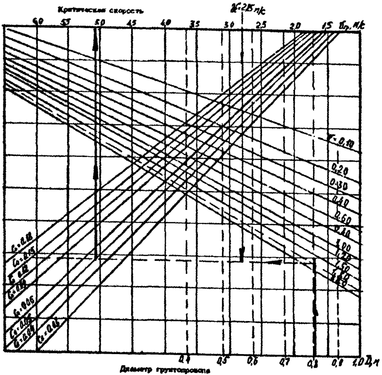
Рис. П.5.2. Номограмма для определения критической скорости смеси: C_o - действительная объемная констигенция смеси, \psi - коэффициент транспортабельности.
