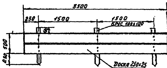
Рис. II. 7.6. Отбойный щиток.
