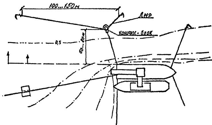
Рис. П 2.2. Леерное устройство на мелководье
