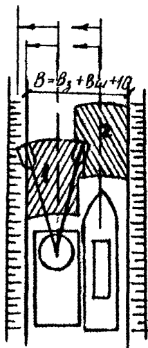
Рис.2. Разработка прорези на мелко-водье и в сухом берегу: B - ширина прорези, B_3 - ширина земснаряда, B_{ш} - ширина шаланды
