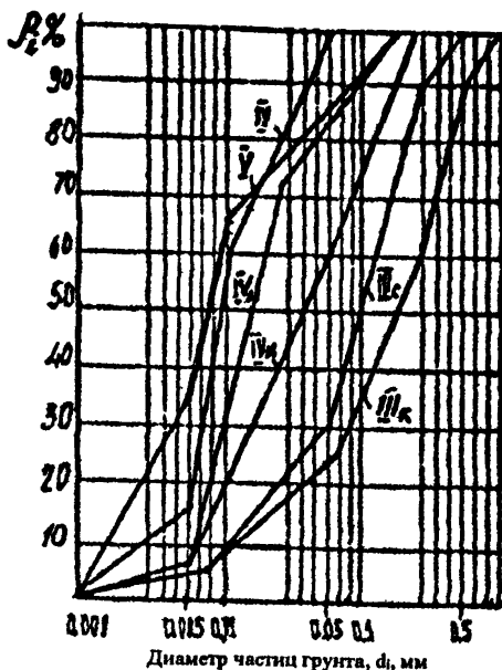
Рис. 14. Гранулометрический состав грунта, ушедшего в перелив
