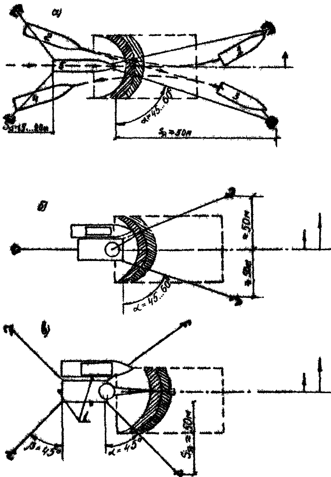
Рис.3. Схемы установки одночерпаковых земснарядов на участке работ а - Схема установки грейферного самоотвозного земснаряда, б - Схема установки грейферного несамоходного земснаряда, в - Схема установки штангового земснаряда, 1 - Сваи
