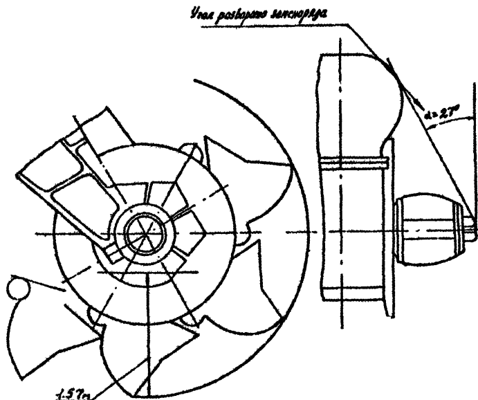
Рис.25. Угол разворота земснаряда при разработке связных грунтов толщиной слоя более 1,60 м у бровки.
