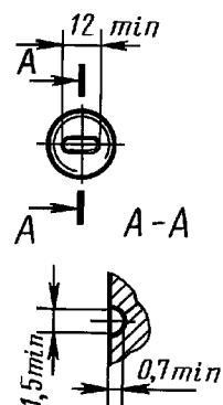
Вариант указательной канавки
