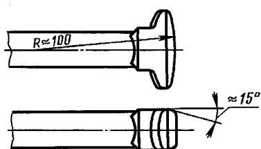
Вариант головки
