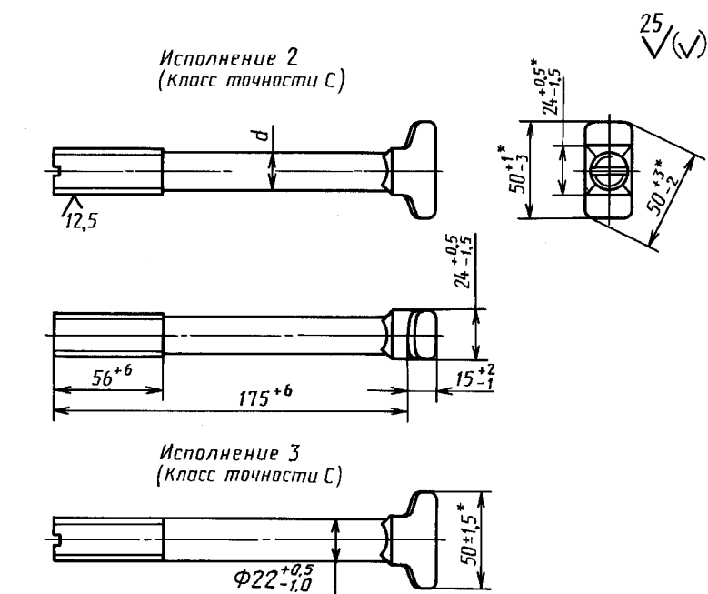
Вариант головки
