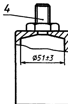
Жидкостная камера с одним отверстием
