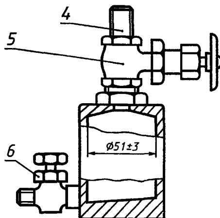
Жидкостная камера с двумя отверстиями
