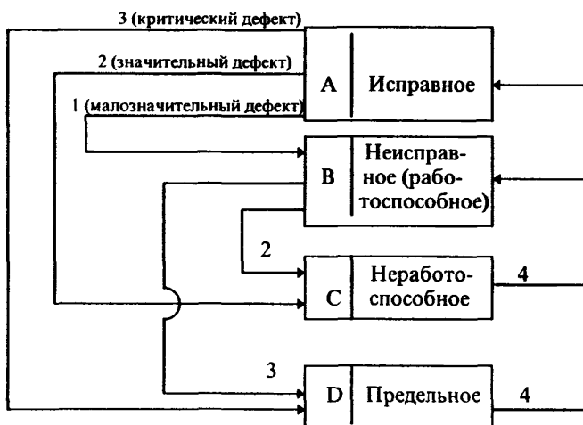
Рис.6.1. Схема основных технических состояний (А, В,С, D) и изменяющих их событий: 1- повреждение, 2- отказ, 3- переход в предельное состояние из-за наличия критического дефекта, 4- ремонт.
