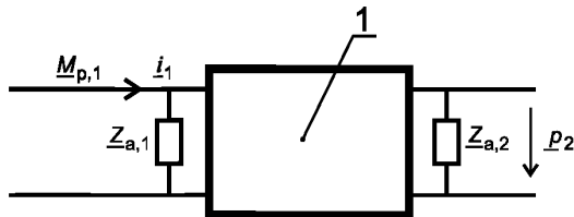
1 — камера связи
