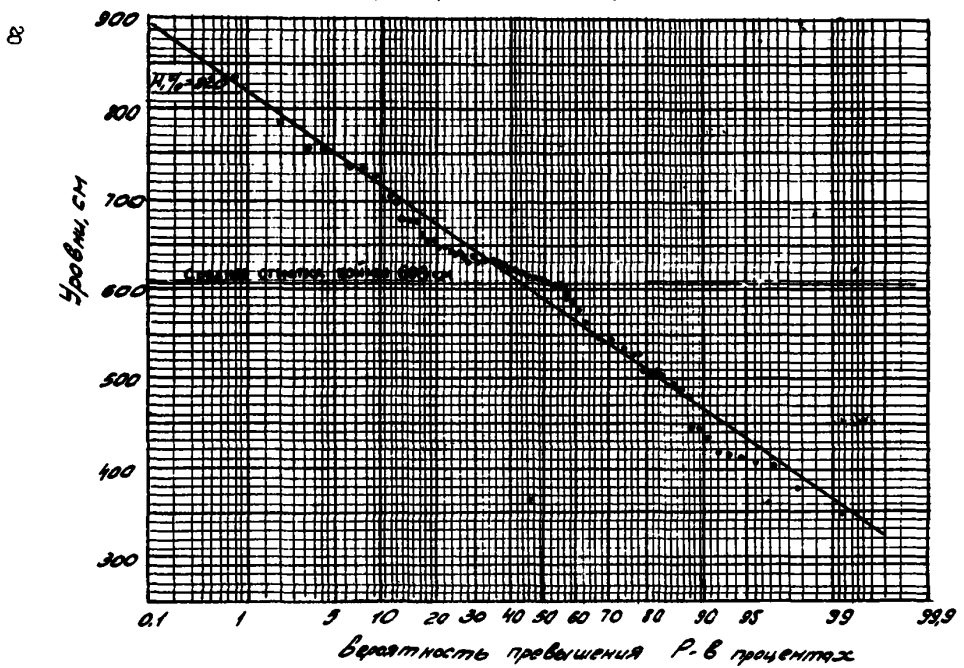
Кривая обеспеченности максимальных уровней воды по ВЛК с 1894 по 1970 гг
