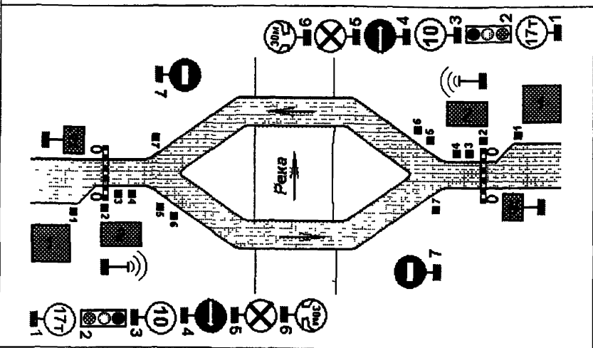
Рис.8.3. Схема организации движения на ледовой переправе при двух отдельных полосах движения для каждого направления 1 - помещение для ожидания и обогрева пассажиров; 2 - контрольно-пропускной пункт, 3 - транспарант "Правила пользования переправой"
