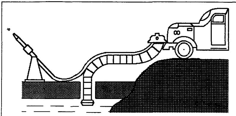
Рис.П.4.3. Намораживающий агрегат "Град-3"
