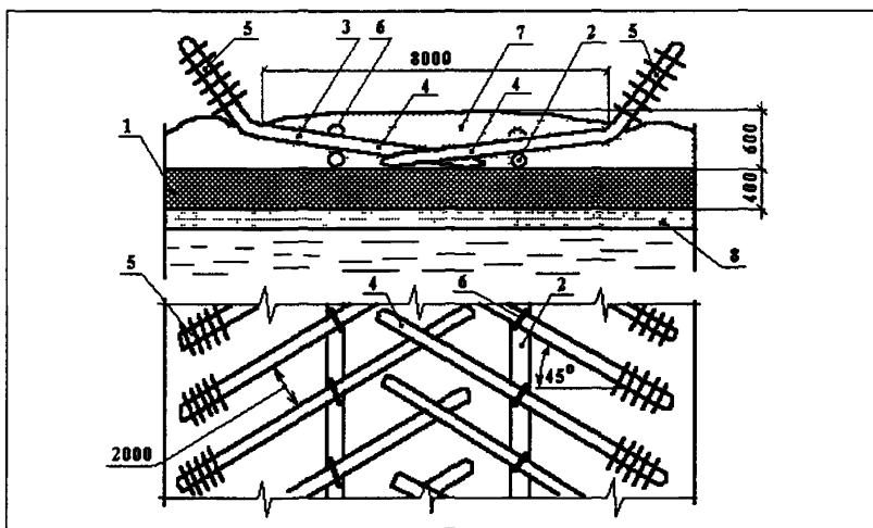
Рис.4.4. Ледовая переправа с теплоотводящими элементами в ледяном покрове 1 - естественный лед, 2 - продольные лежни, 3 - наклонные термосифоны, 4 - испарители термосифонов, 5 - конденсаторы термосифонов, 6 - металлические скобы; 7 - лед, намороженный сверху, 8 - то же, снизу
