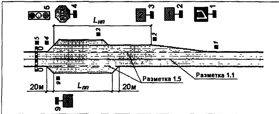
Рис.8.5. Принципиальная схема организации движения на подходе к ледовой переправе в зонах накопительных и посадочных полос 1 - транспарант "Левая полоса для приоритетного движения", 2 - транспарант "Место для высадки пассажиров", 3 - транспарант "Место для посадки пассажиров"
