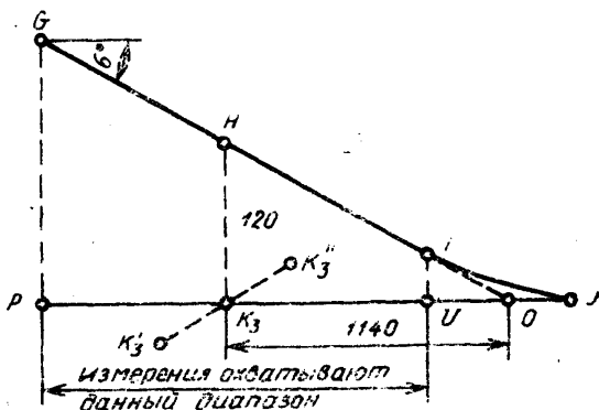
Типичная траектория захода на посадку
