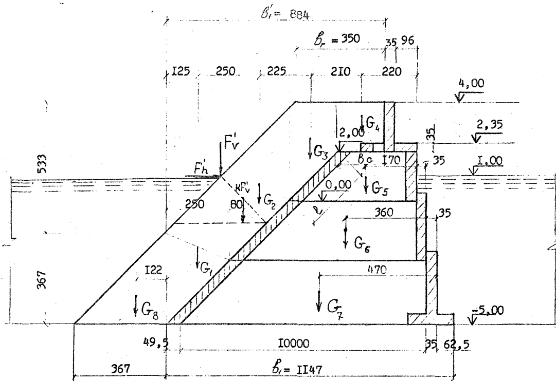
Рис.14. К определению веса элементов конструкции.
