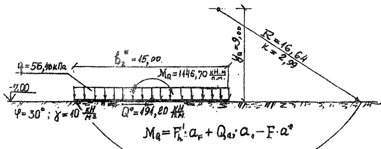
Рис. 19. Расчет общей устойчивости приведенного фундамента.
