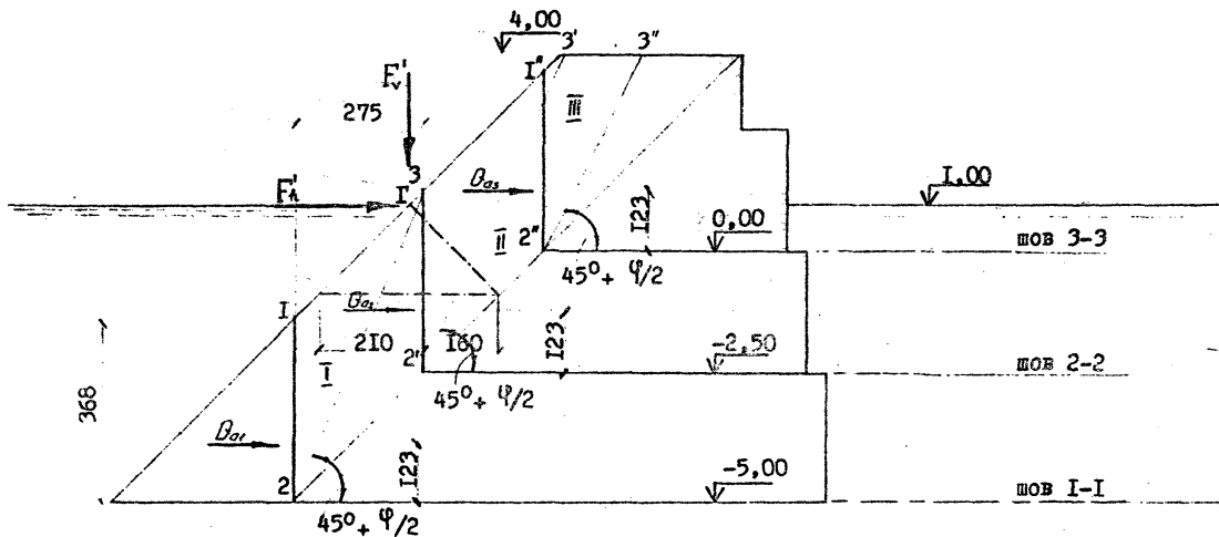
Рис.13. К определению давления льда и наброски при расчете устойчивости на сдвиг по швам конструкции экрана.
