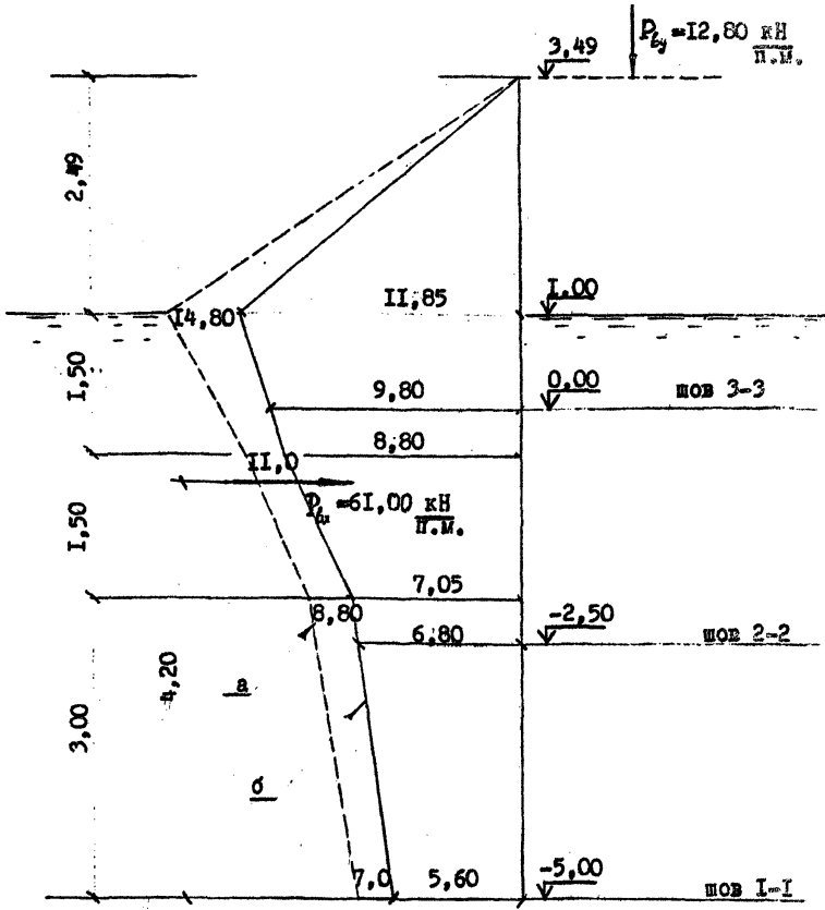
Рис.12. Строительный случай - перфорированная наклонная плита не покрыта тетраподами. Эпиры волнового давления : а) на сплошную вертикальную стенку ; б) на вертикальную плиту экрана и на расчетную плоскость всего сооружения (с учетом коэффициента снижения K_c=0,8 ; интенсивность в кПа)
