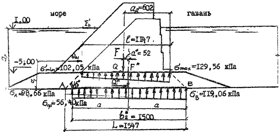
Рис.17. Напряжения з основания и приведенный фундамент.
