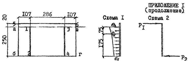
Рис.23. Расчетные схемы вертикальной плиты 2-го курса массивов.
