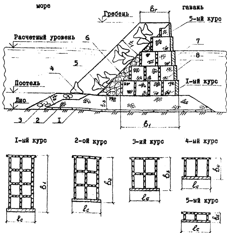
Рис.4. Сооружение с экраном из пустотелых железобетонных массивов, заполненных камнем :
