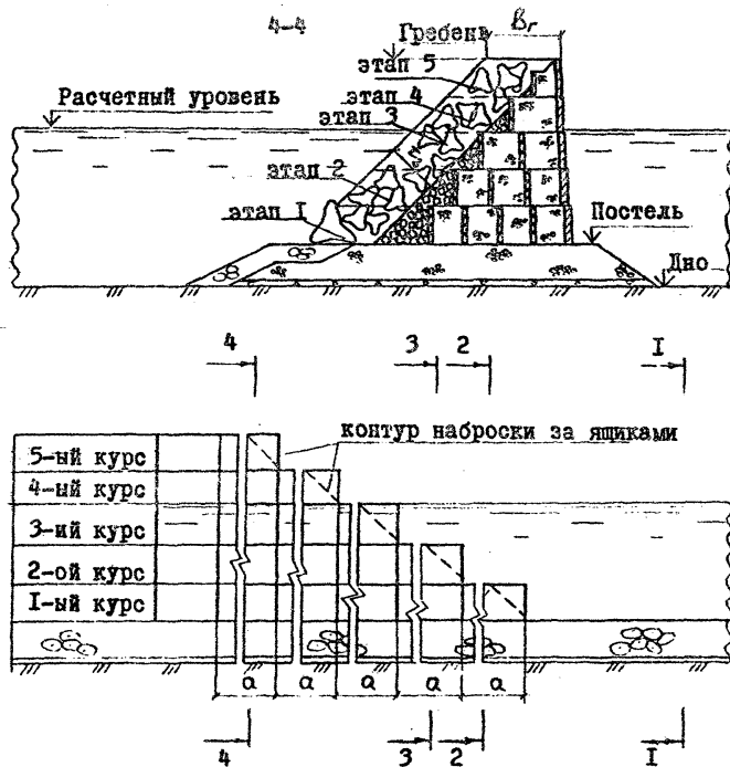
Рис. 9 . Последовательность производства работ
