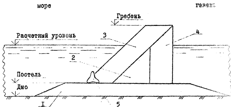
Рис.1. Схема сооружения :
