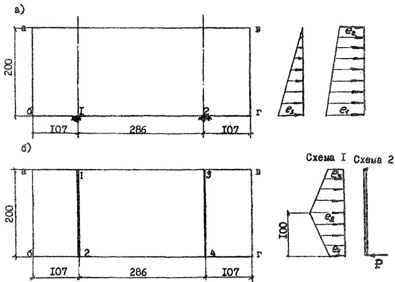
Рис.23. Расчетные схемы вертикальной плиты 2-го курса массивов.
