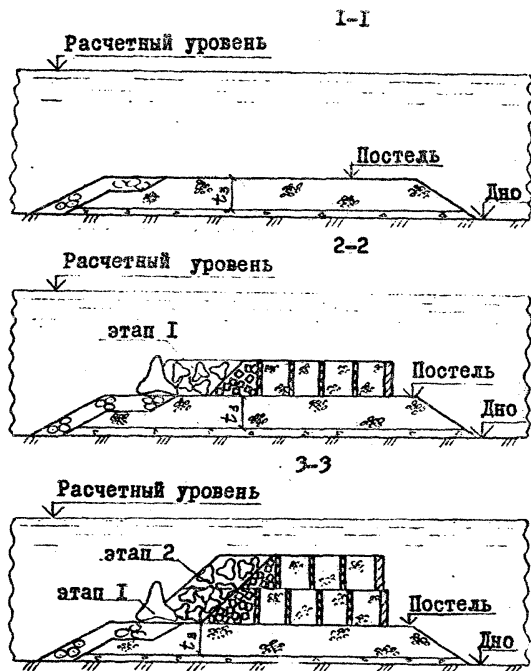
Рис. 9 . Последовательность производства работ
