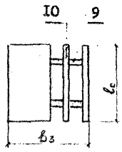
Рис.5. Сооружение с экраном из железобетонных пустотелых массивов с камерой гашения : I - обратный фильтр (щебень, гравий) ; 2 - камень массой 30-100 кг ; 3 - камень крупный массой более 960 кг ; 4 - упорный тетрапод ; 5 - тетраподы ; 6 - железобетонный массив ; 7 - камера гашения ; 8 - железобетонная балка ; 9 - поперечные стенки-рамы ; 10 - рамы-перегородки.
