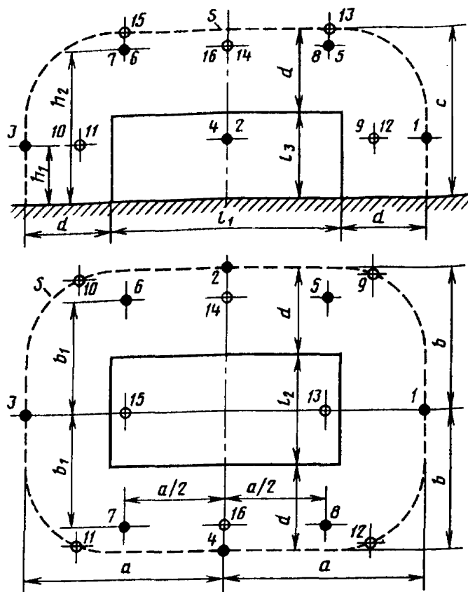
S — измерительная поверхность; 1–8 — точки измерения; 9–16 — дополнительные точки измерения; l_1, l_2, l_3 — размеры огибающего источник шума параллелепипеда; d — измерительное расстояние; a, b, c — характеристические размеры измерительной поверхности
