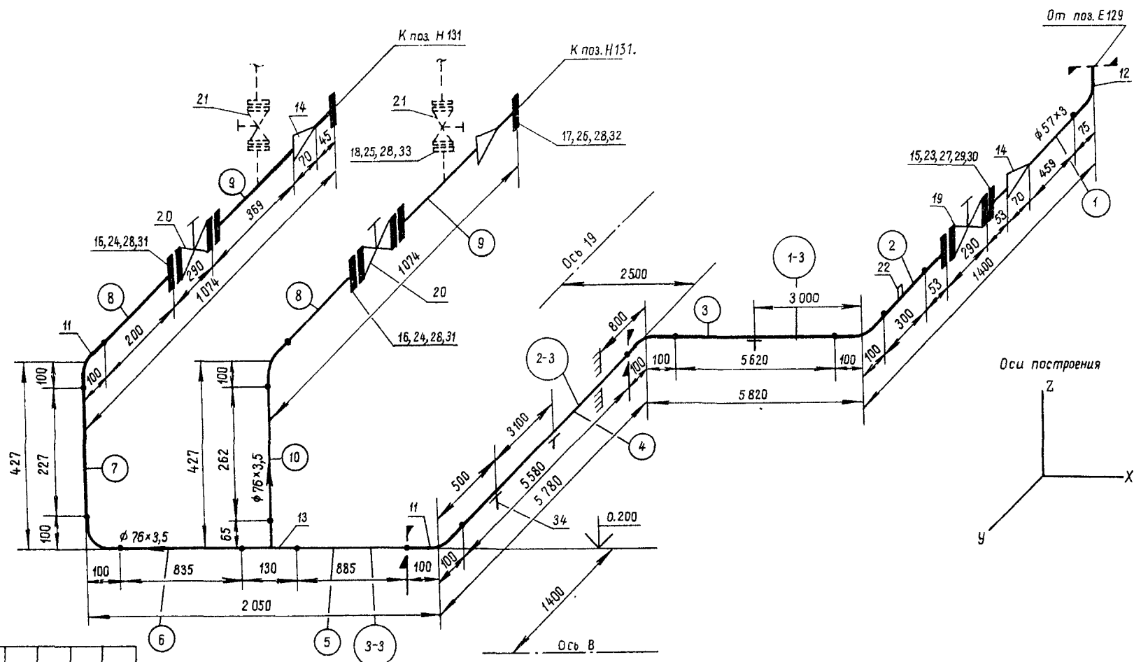
Детализированный чертеж технологического трубопровода, выполняемого с простановкой цепочек размеров
