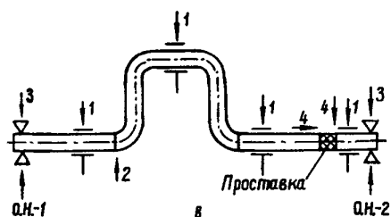
Черт. 15. Последовательность операций (1-5) при монтаже компенсаторов:
