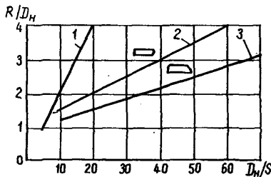
Черт. 6. Определение формы внутреннего дорна:
