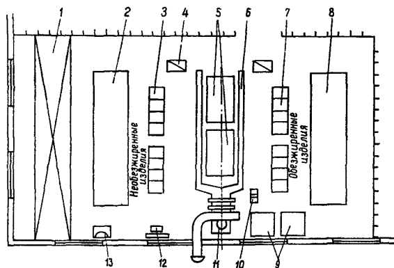
Черт. 19. Схематический план участка обезжиривания:
