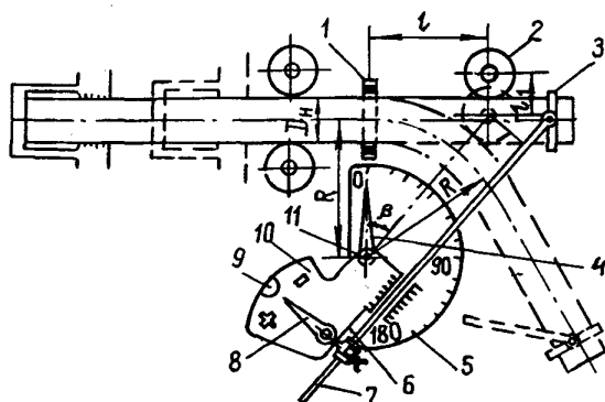
Черт. 9. Схема подготовки станка к работе
