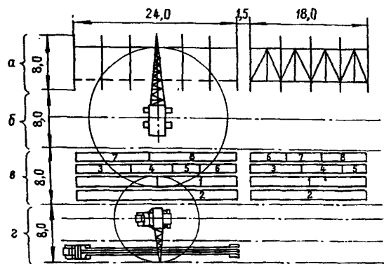
Черт. 17. Схема организации стационарной площадки для сборки блоков строительных конструкций и комбинированных блоков металлических ферменных эстакад:
