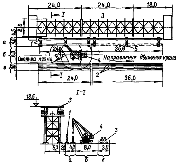
Черт. 16. Схема организации площадки для сборки трубопроводных блоков в зоне действия монтажных кранов:
