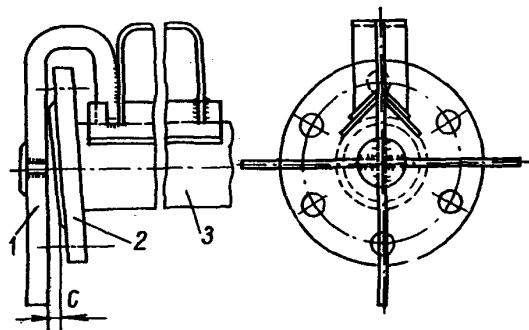
Черт. I3. Контроль отклонения от перпендикулярности уплотнительной поверхности фланца:
