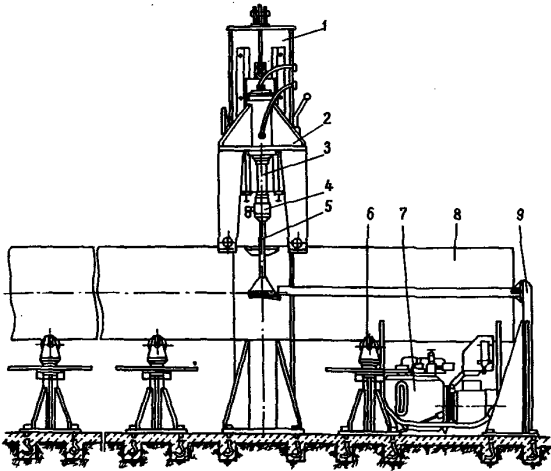
Черт. 3. Установка для вытяжки ответвлений в трубах:
