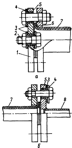
Черт. 22. Конструкция заглушек на конце трубопровода при электролитическом способе испытания:
