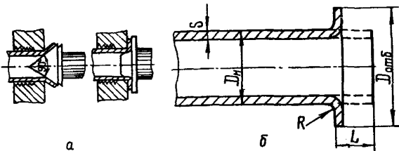
Черт. 2. Отбортовка концов труб (а) и отбортованный конец трубы (б)
