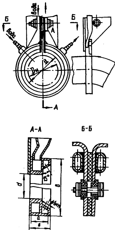
Черт. 8. Двухкамерный индуктор
