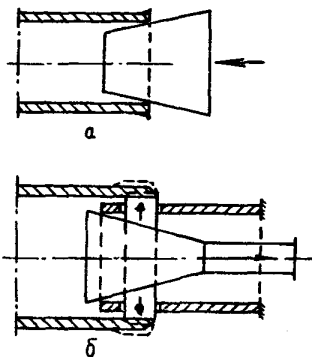
Черт. II. Схемы устройств для калибровки концов труб и деталей трубопроводов:
