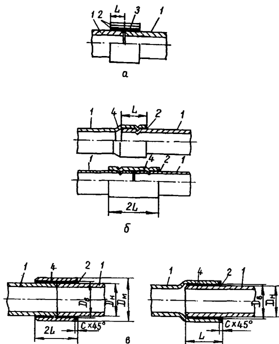
Черт. I4. Схемы клеевого соединения бандажного типа (а), клеємеханического (б) и муфтового (раструбного) (в):
