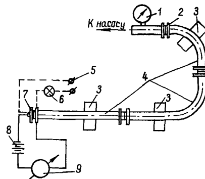
Черт. 21. Принципиальная схема испытаний на сплошность покрытия гуммированного или футерованного трубопровода:
