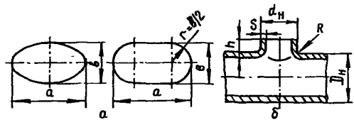
Черт. 4. Форма отверстия (а) для ответвлений в трубах (б)
