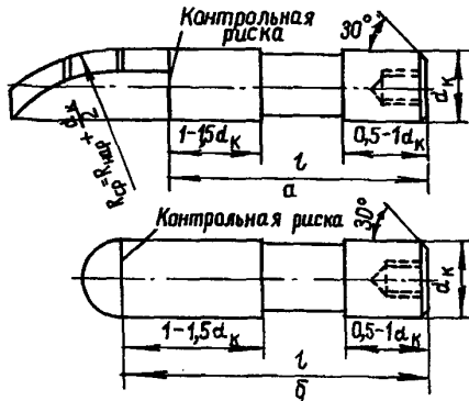
Черт. 5. Стальные дорны: а - ложкообразный; б - шарообразный
