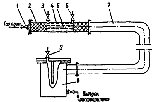
Черт. 18. Схема обезжиривания комбинированным методом:
