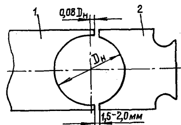
Черт. 7. Зазор между ползуном и гибочным диском:
