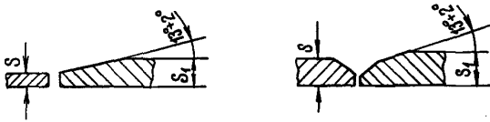
Черт. 1. Форма и размеры скоса кромок при различной толщине свариваемых деталей
