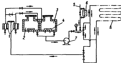
Черт. 20. Принципиальная схема установки для травления трубопроводов растворами ортофосфорной кислоты:
