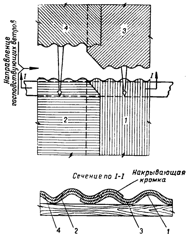
Рис. 7. Способ укладки асбестоцементных волнистых листов без смещения кромок, но со срезкой угол
