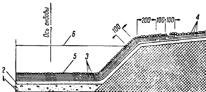
Рис. 2. Оклейка ендовы рулонными материалами и стыкование их слоев со слоями основного ковра на плоскости кровли
