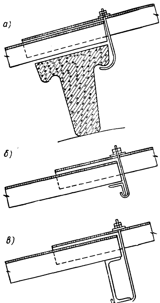
Рис. 8. Крепление асбестоцементных волнистых листов крюками к прогонам а—струннобетонным; б—стальным прутково-шпренгельным; в—стальным шпренгельным
