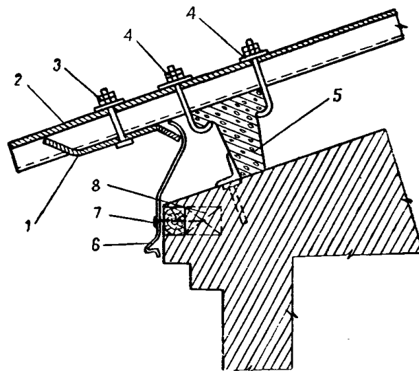
Рис. 9. Устройство кровли из асбестоцементных волнистых листов на карнизе
