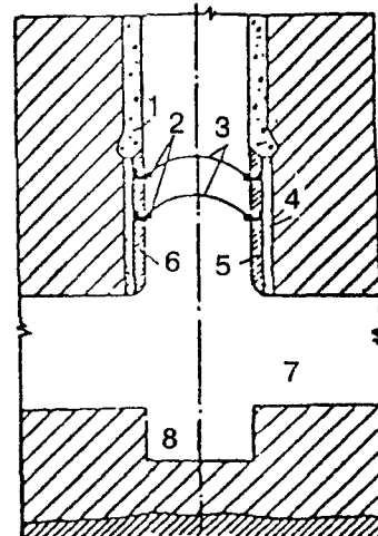
1 — опорный венец крепи ствола; 2 — кольцевые металлические воротники; 3 — металлические перемышки; 4 — продуктонепроницаемый раствор; 5 — металлическая сварная обечайка; 6 — железобетонная рубашка; 7 — выработка-емкость; 8 — зумпф
