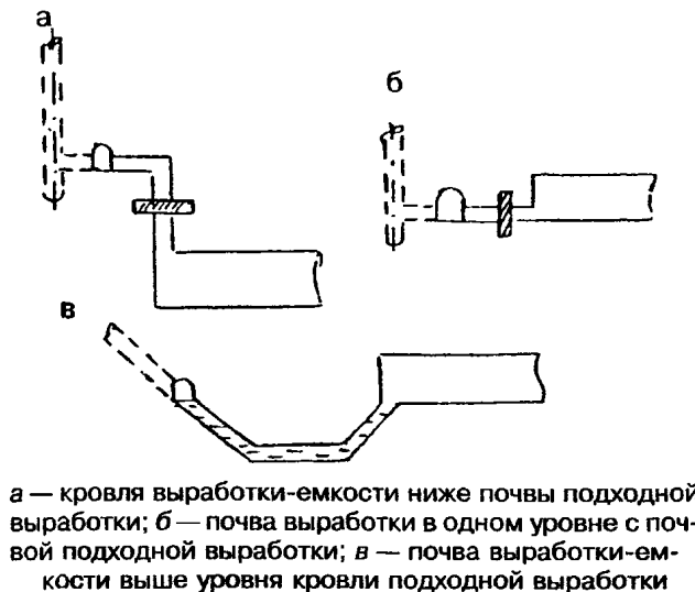
Рисунок 5 — Узел герметизации выработок-емкостей
