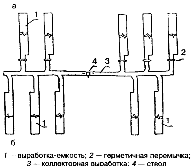
Рисунок 4 — Выработки-емкости для нескольких видов продукта (а) и для одного вида продукта (б)
