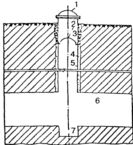
1, 2 — металлические перемышки в обсадной трубе; 3 — устье ствола; 4 — продуктонепроницаемый раствор; 5 — обсадная труба; 6 — выработка-емкость; 7 — зумпф
