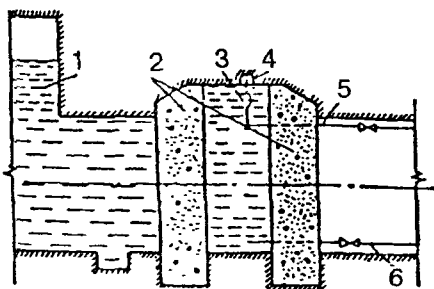
1 — выработка-емкость; 2 — напорные стенки герметичной перемышки; 3 — полость гидрозатвора с изолирующей жидкостью; 4 — штроба; 5 — трубопровод для выпуска воздуха из гидрозатвора; 6 — трубопровод для заполнения гидрозатвора
