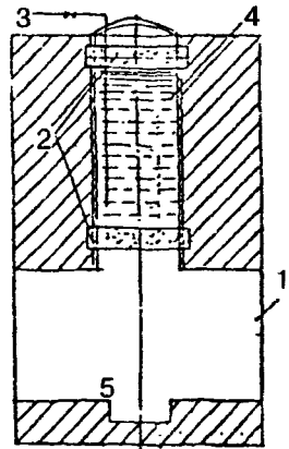
1 — выработка-емкость; 2 — бетонные стенки герметичной перемышки; 3 — трубопровод для заполнения гидрозатвора; 4 — полость гидрозатвора с изолирующей жидкостью; 5 — зумпф
