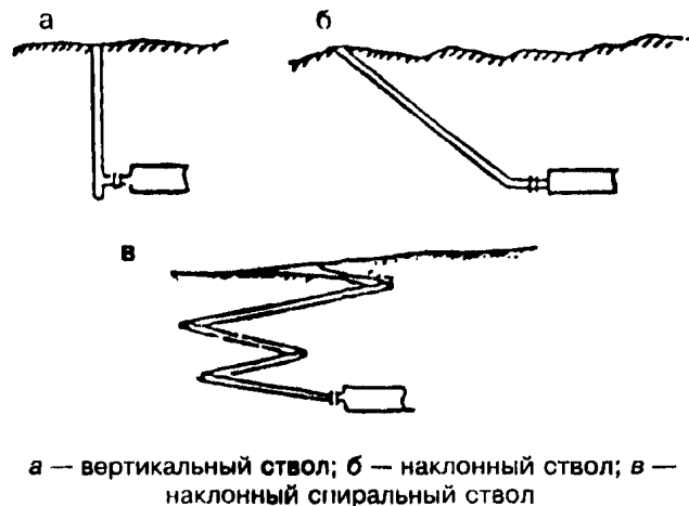
Рисунок 3 — Вскрывающие выработки
