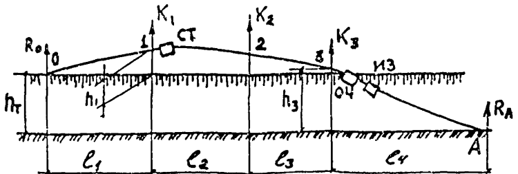
Расчетно-технологическая схема
