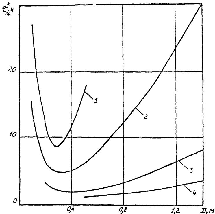
Рис.2. Зависимость времени прокачки воды с температурой T_B^* = 50^\circ\text{C} для эталонного трубопровода от его диаметра при суммарной производительности наполнительных агрегатов Q , \text{м}^3/\text{ч} :
