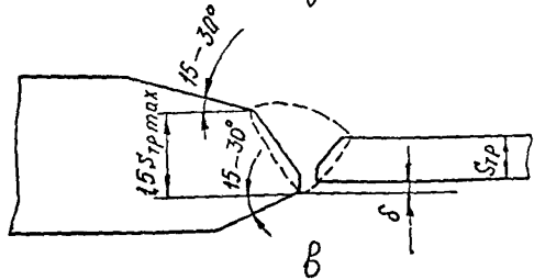
Рис.2. Варианты сборки стыков разнотолщинных элементов: а - совпадение наружных диаметров трубы и детали; б - совпадение внутренних диаметров; в - сборка разнотолщинных элементов при несопадении диаметров; S - номинальная толщина стенки детали; S_{тр} - нормативная толщина стенки трубы; \delta - смещение кромок при сборке стыка; D_{тр} - наружный нормативный диаметр трубы; D_{сд} - сборочный диаметр D_{сд} = (D_{тр} - 2S_{тр}) \pm 1 мм
