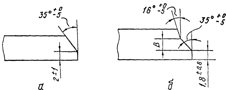
Рис. I. Формы подготовленных кромок:
