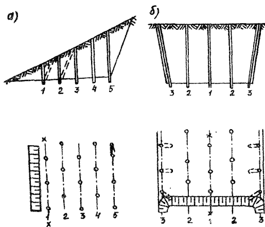
Рис. 5. Продольно-порядные схемы КЗВ: a — для выемки на косогоре; b — для выемки на равнинном участке; 1, 2, 3, 4, 5 — очередность взрывания рядов скважин
