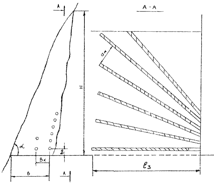
Рис. 20. Схема взрыва на обрушение вертикальными скважинами
