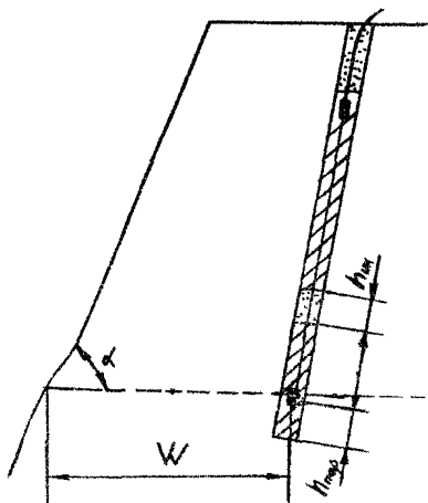
Рис. 16. Конструкция заряда в скважинах первого ряда
