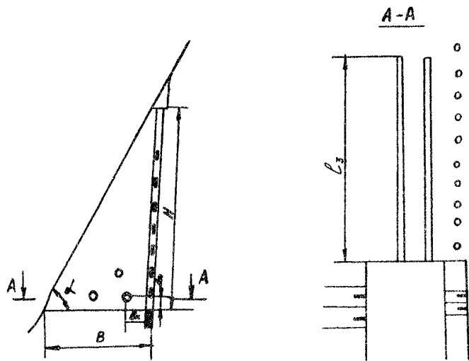
Рис. 19. Схема взрыва на обрушение горизонтальными скважинными зарядами
