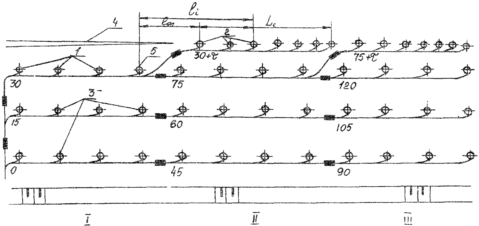
Рис. 34 Схема контурного взрывания способом КВИН: 1—скважины предконтурного ряда; 2—контурные скважины; 3—скважины рыхления; 4—контурная щель; 5—ближайшая скважина предконтурного ряда; I, II, III—зоны секций
