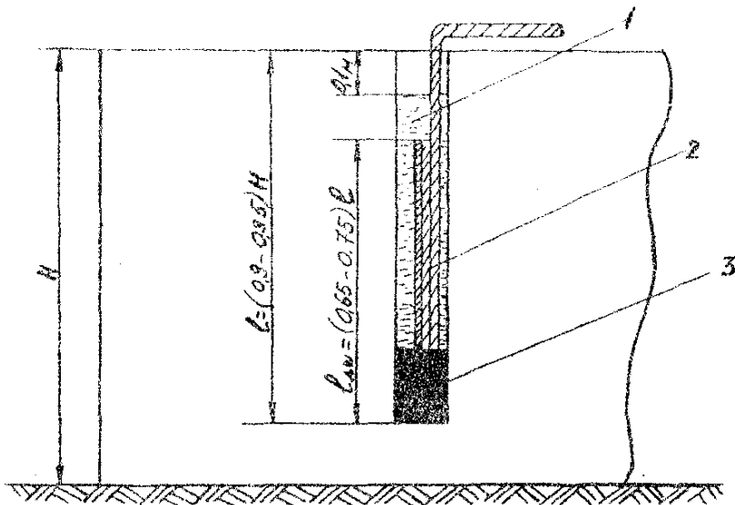
Рис. 30. Конструкция заряда при гидровзрывном способе разрушения фундаментов: 1—вода в шнуре; 2—нити ДШ; 3—дополнительный заряд ВВ
