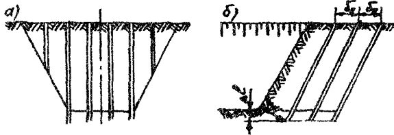
Рис. 4. Схема расположения скважин в неустойчивых породах при лобовой разработке выемки:
