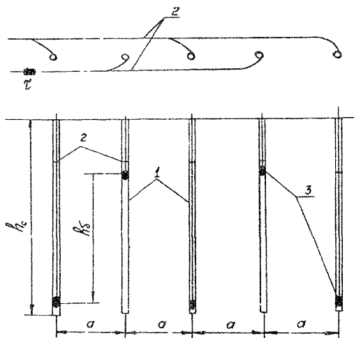
Рис. 35. Схема инициирования контурного ряда скважинных зарядов способом ВИСС (с помощью ДШ).
