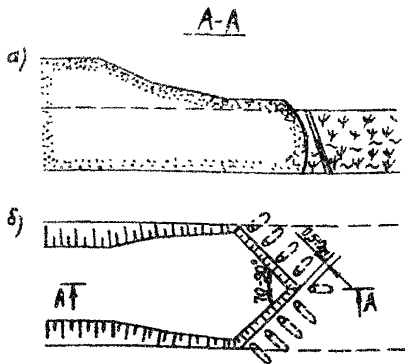
Рис. 26. Схема расположения зарядов при образовании поперечных траншей в «голове» насыпи:
