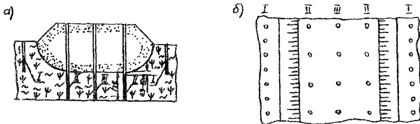
Рис. 27. Схема расположения скважинных зарядов в разрезе (а) и плане (б) при посадке насыпи на минеральное дно болота:
