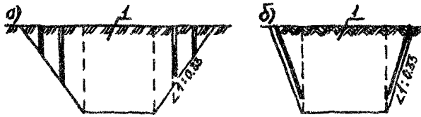
Рис. 2. Расположение вертикальных (а) и наклонных (б) откосных скважин в поперечном профиле выемки:
