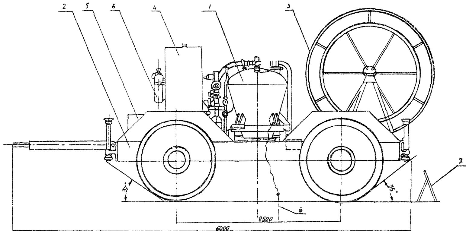
Рис 38. Транспортно-зарядная установка ТЗУ-Т
