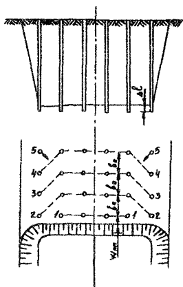
Рис 6 Поперечно-порядковая схема КЗВ
