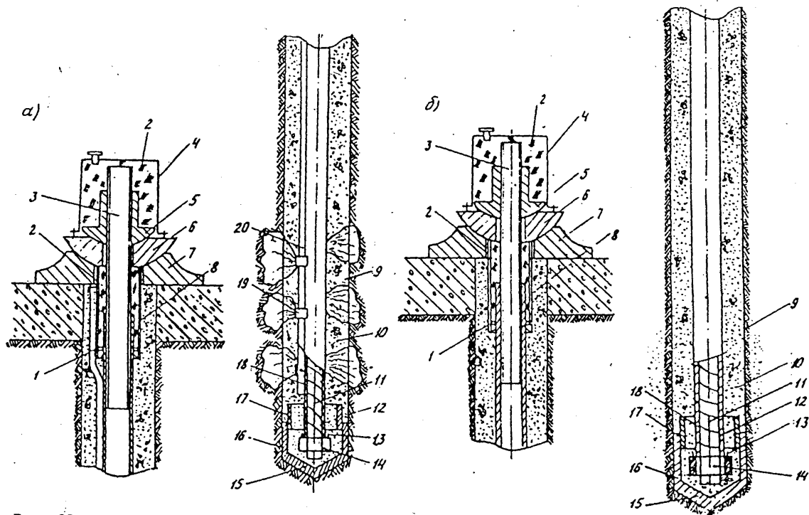
Рис. 22. Грунтовый инъекционный анкер с буровым наконечником для грунтов: а - связных, б - песчаных
