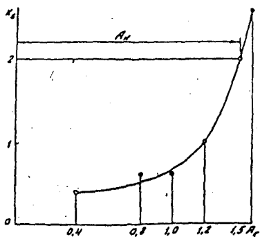
Рис. 28. Пример определения предельной нагрузки
