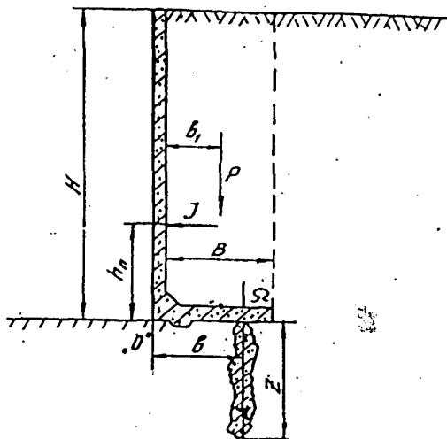
Рис. 36. Схема к расчету сборных подпорных стен, заанкеренных в основании
