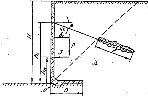
Рис. 35. Схема к расчету сборных заанкеренных подпорных стен
