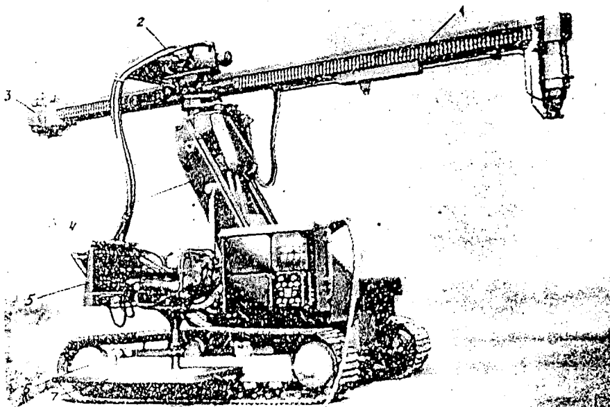
Рис. 4. Универсальный буровой станок: 1 - лафет; 2 - гидроударник; 3 - клещевой захват; 4 - стрела; - пульт управления; 6 - шасси; 7 - подножка оператора
