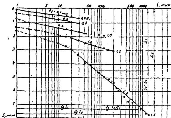
Рис. 27. Графики зависимости деформации во времени для определения коэффициента ползучести: ---- прямойный участок графика, на котором определяется коэффициент ползучести K_s ; --- криволинейный участок графика
