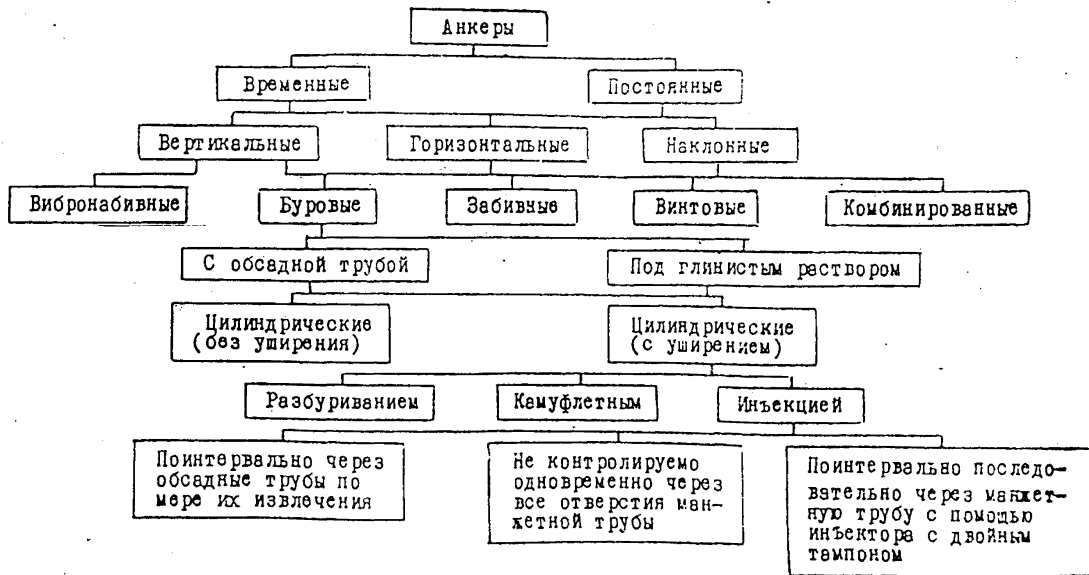
Рис. 2. Классификация анкеров
