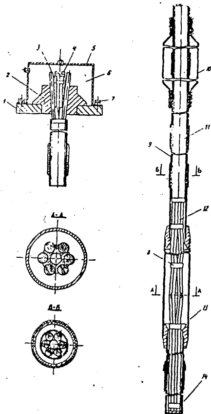
Рис. 20. Грунтовый инъекционный анкер с манжетной трубой при внутреннем расположении тяги
