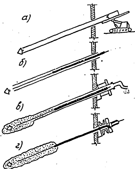
Рис. 24. Технология устройства анкеров "Бауэр"
