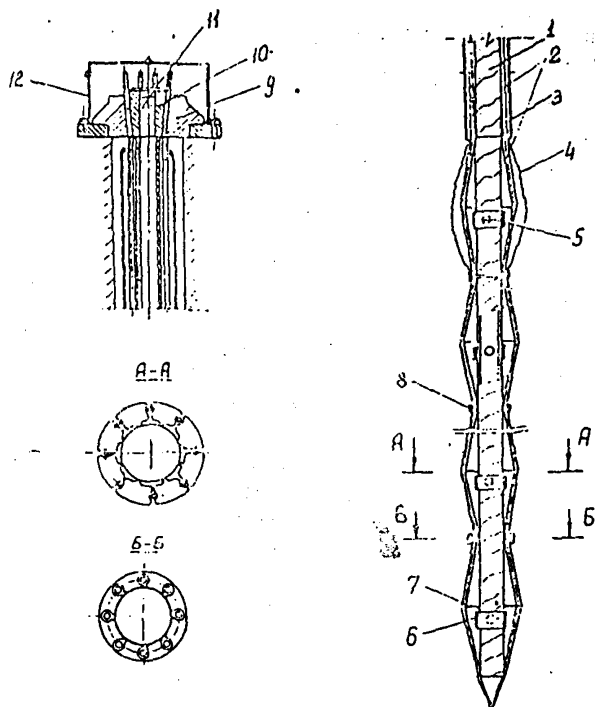
Рис. 14. Временный грунтовый инъекционный анкер с манжетной трубой при наружном расположении неизолируемой тяги
