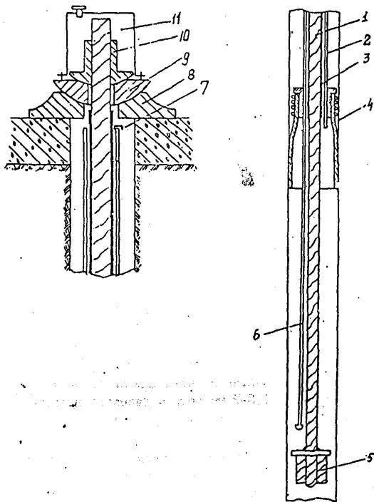
Рис. 15. Временный грунтовый инъекционный анкер с резиновым обтирателем
