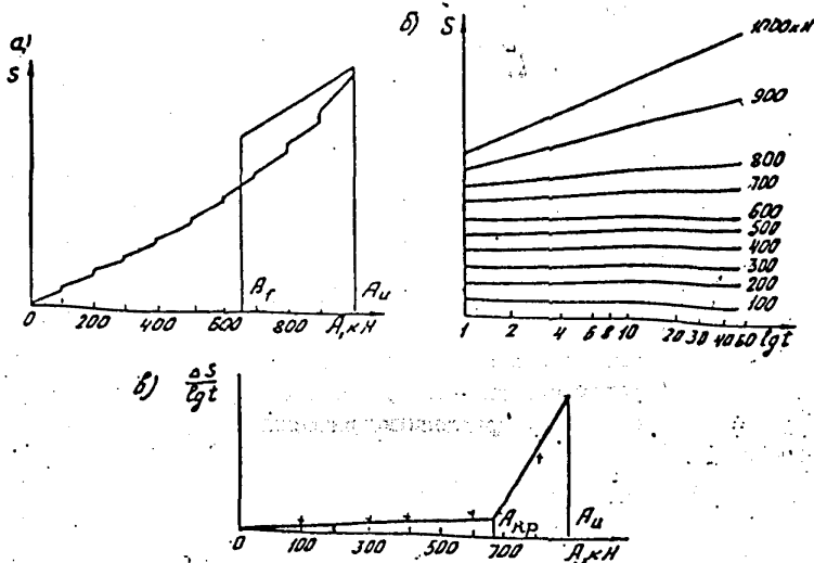
Рис. 30. Графики результатов испытаний:
