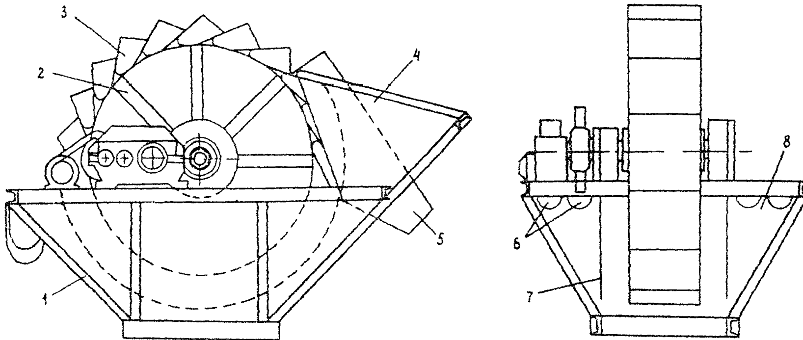
Схема ковшевого классификатора-сбесвозмивателя: 1 - вала, 2 - электродвигательное колесо; 3 - перфорированные ковши; 4 - загрузочная воронка; 5 - точка; 6 - сливные желоба; 7 - перегородки; 8 - боковые отсеки
