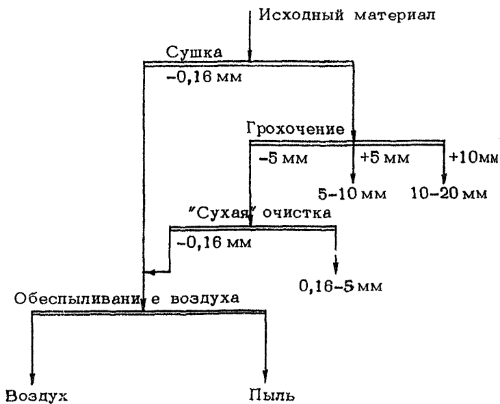
Рис. 7. Технологическая схема "сухого" обогащения влажных отсевов дробления
