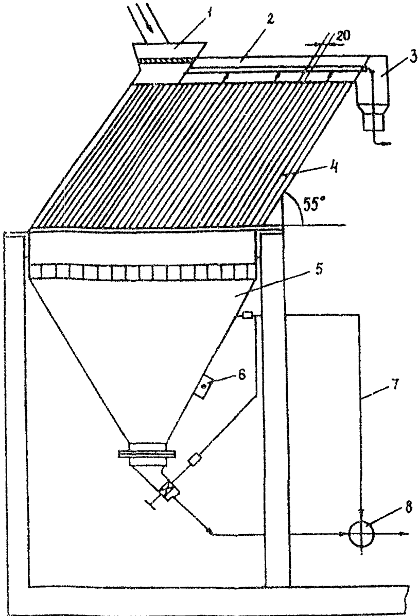
Схема тонкослойного отстойника 1 - приемная воронка; 2 - камера осветления; 3 - патрубок для слива осветленной воды; 4 - пластины; 5 - бункер для сгущенного осадка; 6 - вибратор; 7 - система автоматизированного контроля за уровнем осадка включением и выключением насоса, 8 - насос
