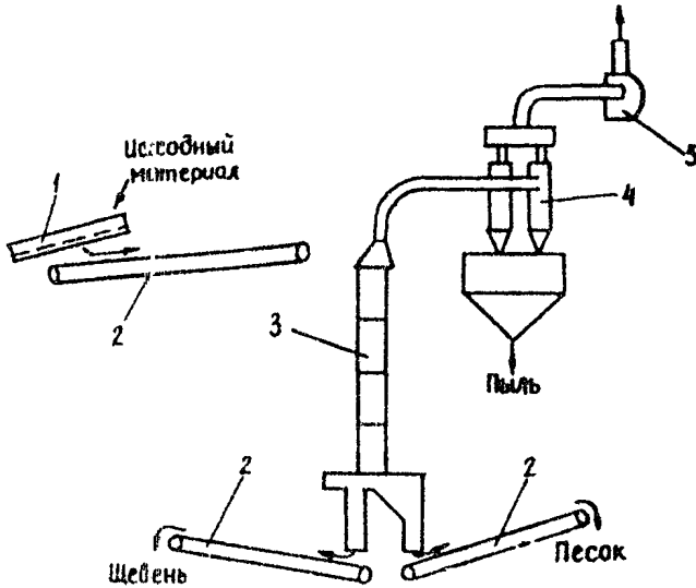
Рис.4. Схема технологической линии ВНИИчеруды для переработки отсевов дробления "сухим" способом: 1 - виброгрохот; 2 - ленточные конвейеры; 3 - вертикальный пневмокласификатор; 4 - циклон; 5 - вентилятор
