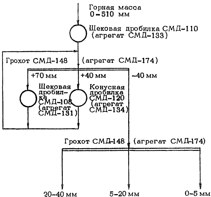
Рис. 4. Технологическая схема переработки каменных материалов на ПДСУ-85
