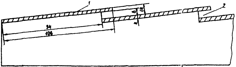
Рис. 3. Уступообразное днище: 1 – пластина; 2 – проем для воздуха
