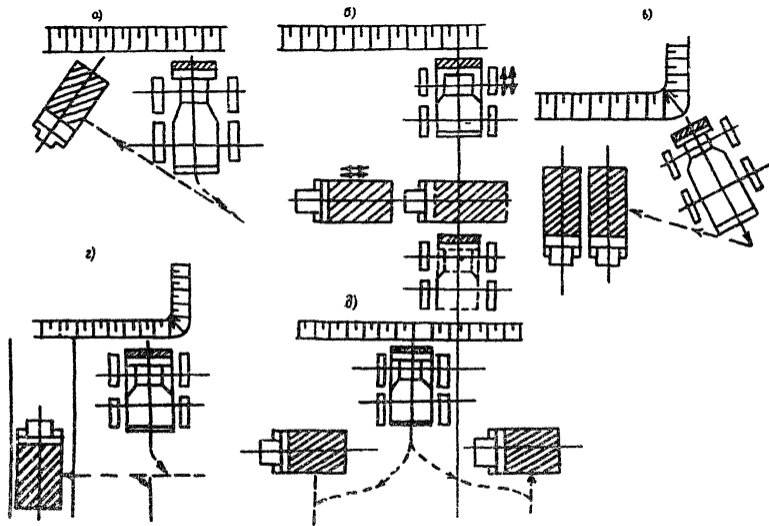
Рис. 2. Схема работы поддежка
