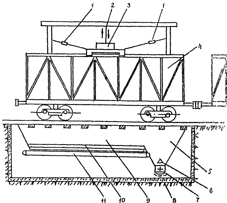
Рис. 12. Схема разгрузки с использованием виброплиты и шелевого бункера: 1 - расчалки с амортизаторами; 2 - подвеска накладной виброплиты; 3 - накладная виброплита; 4 - полувагон; 5 - основной бункер; 6 - вставка основного бункера; 7 - комкорыхлитель; 8 - вывесной конвейер; 9 - шелевой бункер; 10 - вставка шелевого бункера; 11 - подшелевой конвейер
