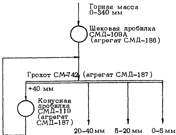
Рис. 3. Технологическая схема переработки каменных материалов на ПДСУ-35
