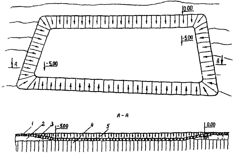
План карьера после рекультивации земель: 1 - растительный грунт, естественный, 2 - песок, 3 - растительный грунт, насыпной; 4 - суглинок. 5 - откос карьера после рекультивации
