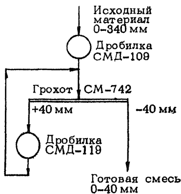
Рис. 9. Технологическая схема производства готовых смесей на ПДСУ-35
