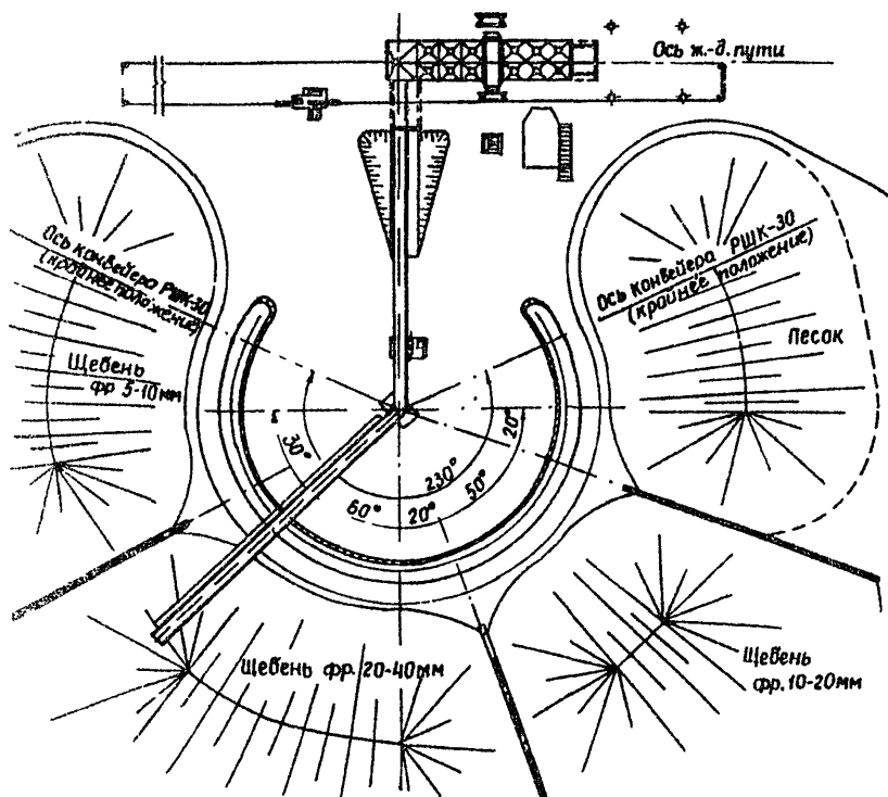
Рис.13. Схема склада нерудных материалов вместимостью 18 тыс.м 3
