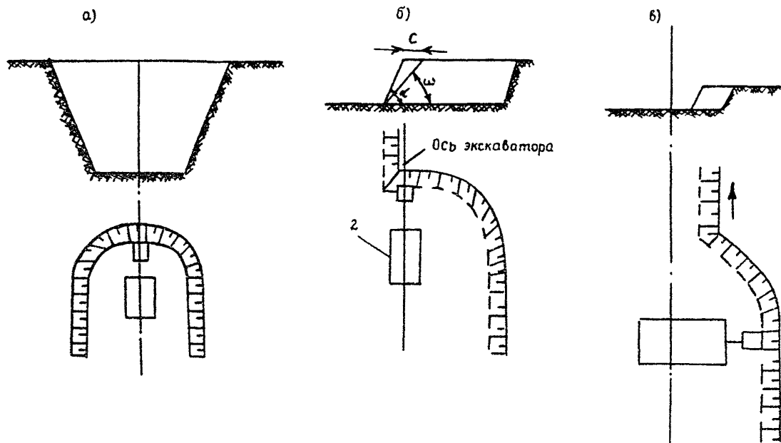
Рис.1. Схема работы экскаватора с прямой лопатой с забоем: а - тупиковым; б - боковым; в - фронтальным: 1 - забой; 2 - экскаватор; \alpha - угол откоса рабочего уступа; \omega - угол устойчивого откоса уступа траншеи, с - объем снимаемого материала
