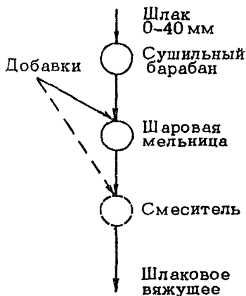
Рис. 14. Схема получения шлакового вяжущего
