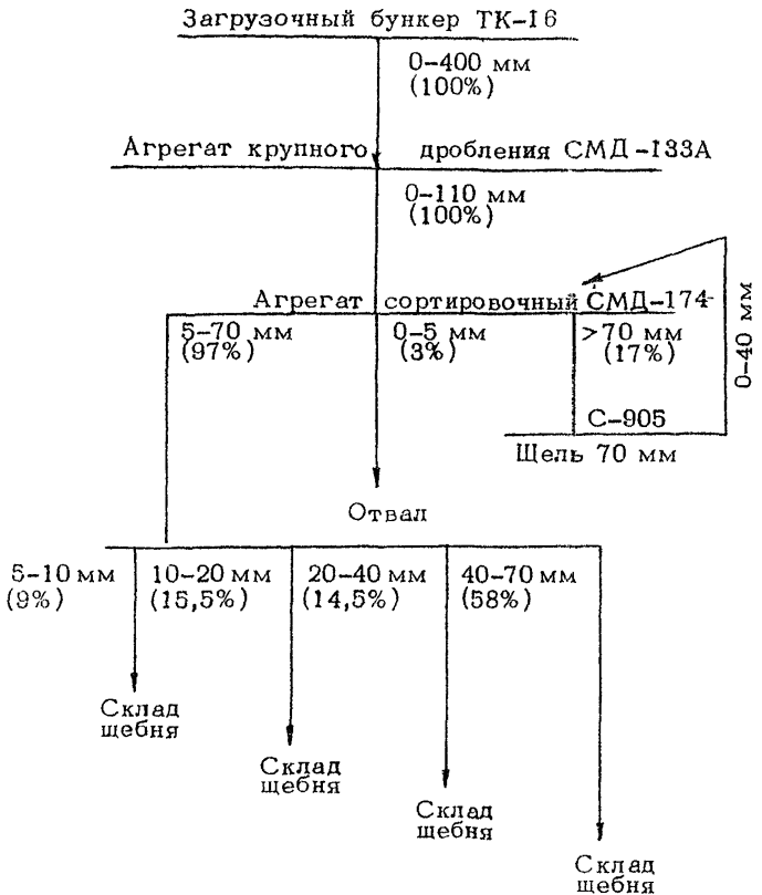
Схема технологического процесса дробления
