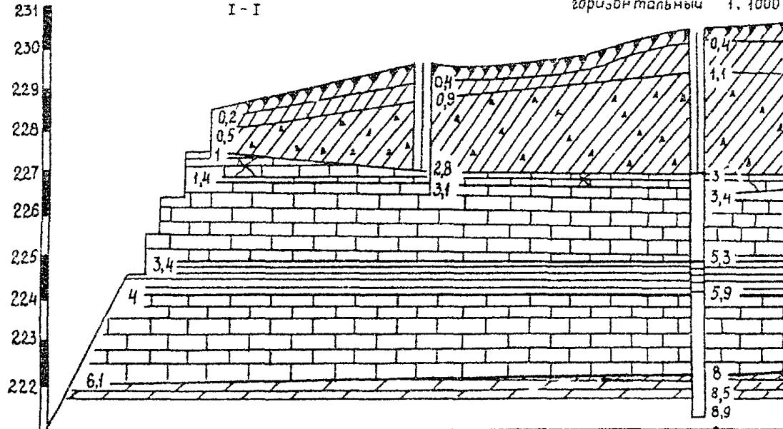
Геолого литологический разрез
