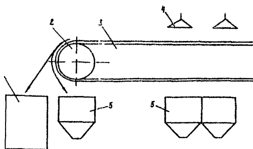
Рис.15. Схема удаления металла из металлургических шлаков: 1 - дробилка; 2 - электромагнитный шкив; 3 - ленточный конвейер; 4 - подвесные электромагниты; 5 - бункер для сбора металла
