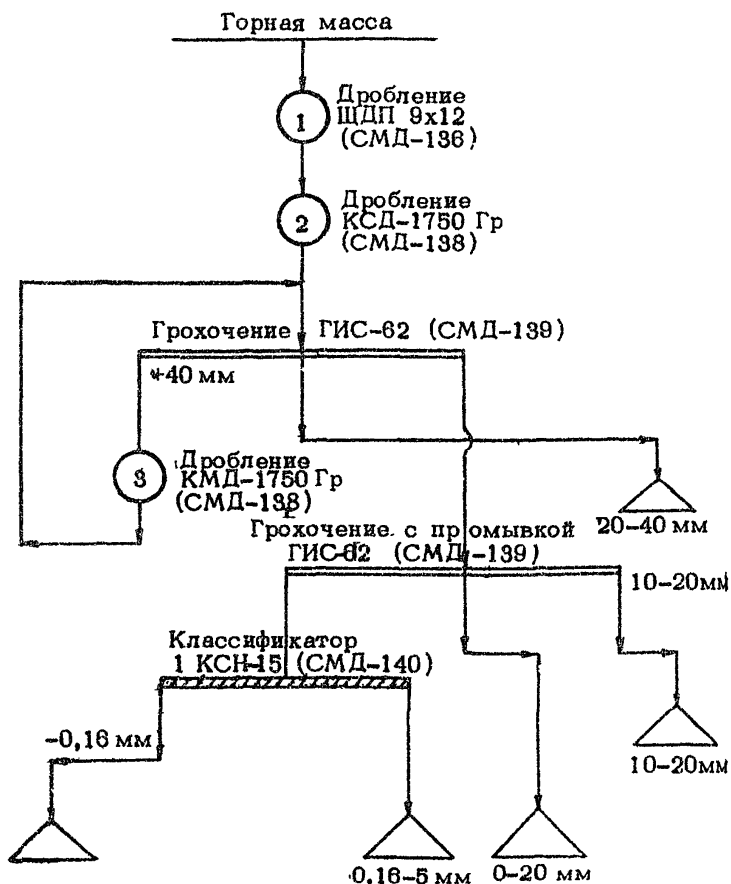
Рис. 5. Сборно-разборная дробильно-сортировочная автоматизированная линия САДЛ-И-400
