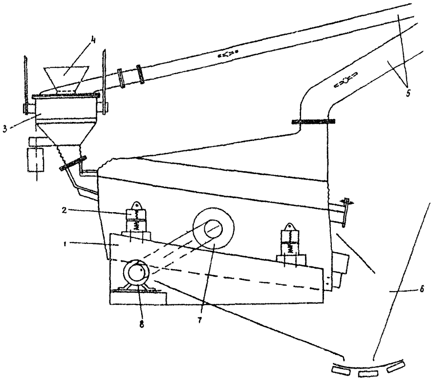
Рис.1. Общий вид виброочистителя песчаных материалов: 1 - виброгрохот; 2 - пружина; 3 - дезинтегратор; 4 - загрузочная воронка; 5 - воздуховоды; 6 - приемный лоток; 7 - вибратор; 8 - электродвигатель
