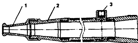
Рис. 2.1. Ствол-водомер: 1 - насадка мерный; 2 - ствол в сборе; 3 - штуцер для манометра
