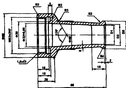
Рис. 2.1. Ствол-водомер: 1 - насадка мерный; 2 - ствол в сборе; 3 - штуцер для манометра
