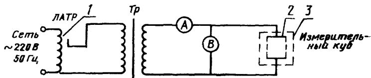
1—лабораторный регулировочный трансформатор (ЛАТР); 2—электрод; 3—измерительный куб
