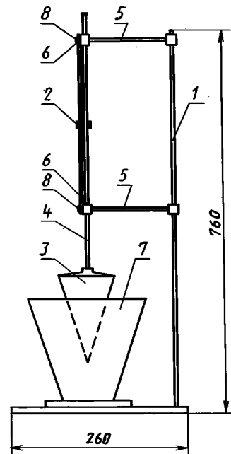
Прибор для определения подвижности растворной смеси
