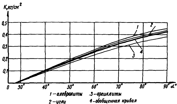
Рис.1. Графики зависимости критической прочности пород слоистой толщи - аргиллитов, алевролитов и углей - от угла откоса уступа (Богославский карьер)
