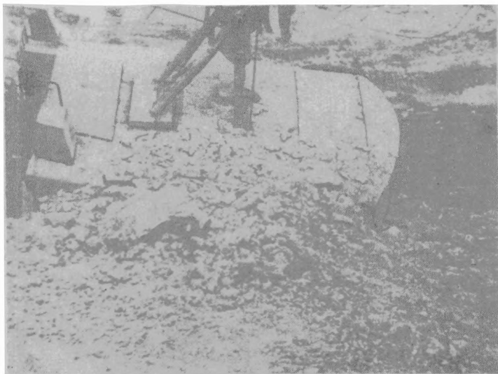
Рис.3. Обрушение уступа 17 августа 1967 года на карьере "Миллионный"
