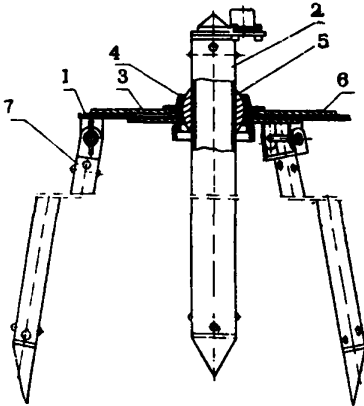
Рис.1. Жесткий отвес ОЖ-3
