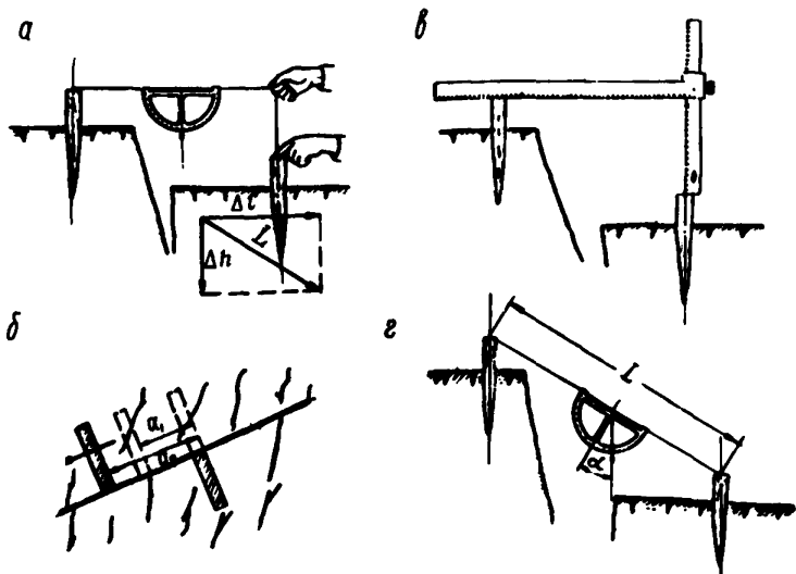
Рис.8. Наблюдения за развитием заделов и трещин а,г—измерения с применением шпагата и угломера; б—наблюдения за смещением массива по поверхности ослабления с применением маркирующих штрихов; в—измерения с использованием оцинкованных реек
