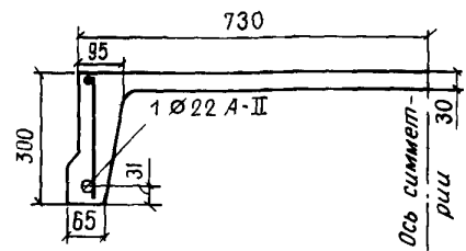
Черт. 89. К примеру расчета 59
