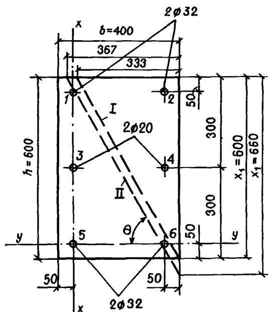
Черт. 50. К примерам расчета 38 и 40
