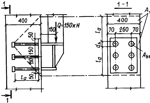
Черт. 77. К примеру расчета 50
