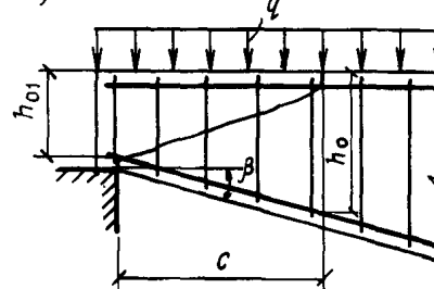
Черт. 18. Балки с переменной высотой сечения и наклонной гранью
