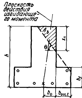
Черт. 8. Тавровое сечение со сжатой зоной, заходящей в наименее растянутый свес полки
