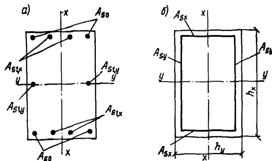
Черт. 43. Схемы расположения арматуры в прямоугольном сечении при расчете на косое внецентренное сжатие
