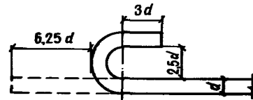
Черт. 92. Размеры крюков на концах стержней гладкой ребочей арматуры
