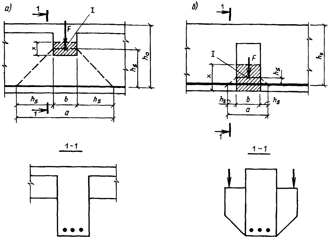
Черт. 66. Схема для определения длины зоны отрыва
