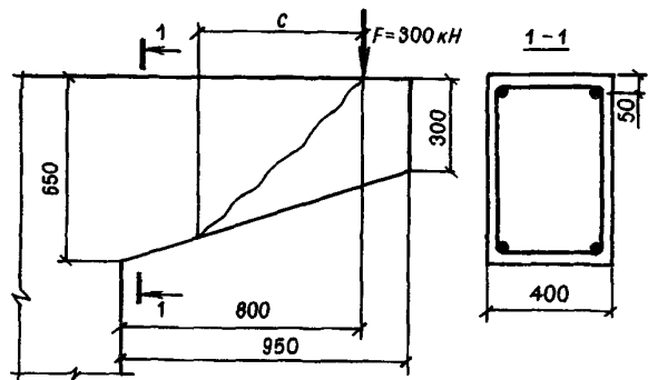
Черт. 29. К примеру расчета 18
