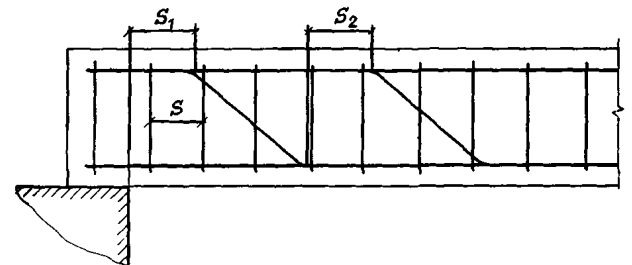
Черт. 12. Расстояния между хомутами, опорой и отгибами
