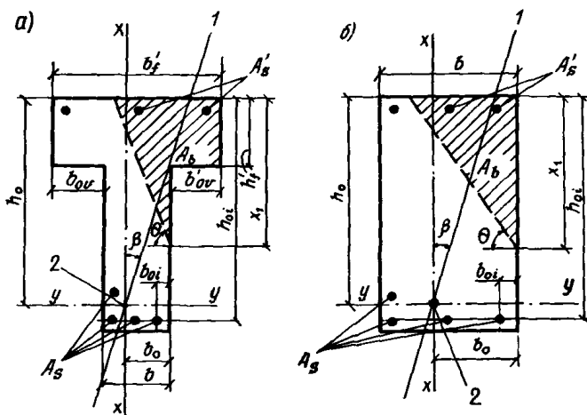
Черт. 6. Форма сжатой зоны в поперечном сечении железобетонного элемента, работающего на косою изгиб
