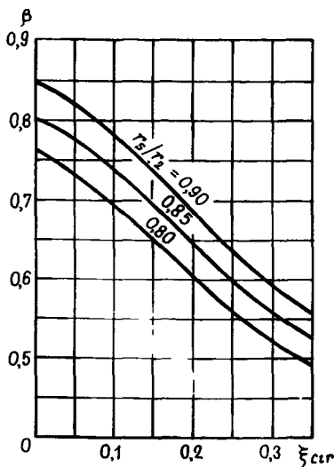
Черт. 60. График для определения коэффициента \beta при расчете элементов кольцевого поперечного сечения на кручение с изгибом
