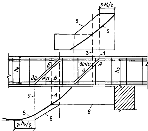
Черт. 116. Положения отгибов, определяемые опорой изгибающих моментов в балке
