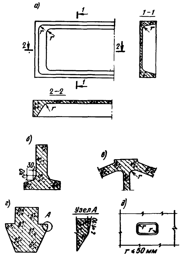
Черт. 90. Закругления и фаски
