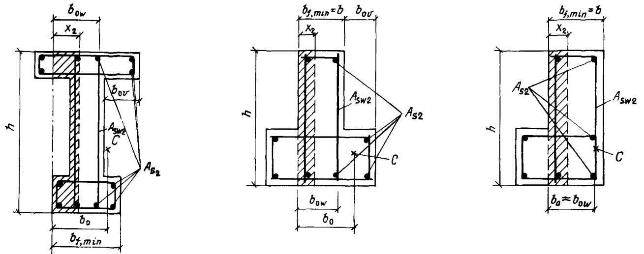
Черт. 58. Схемы расположения сжатой зоны в пространственном сечении 2-й схемы железобетонного элемента двутаврового, таврового и Г-образного сечений, работающего на кручение с изгибом
