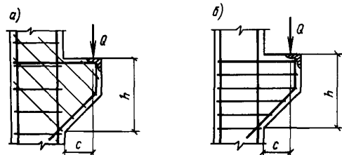
Черт. 118. Короткие консоли колонн с хомутами а — наклонными; б — горизонтальными
