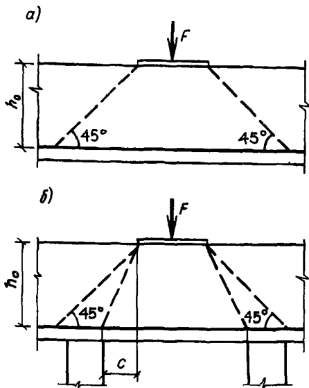
Черт. 65. Схема пирамиды продавливания при угле наклона ее боковых граней к горизонтали a = 45^\circ ; b – более 45^\circ
