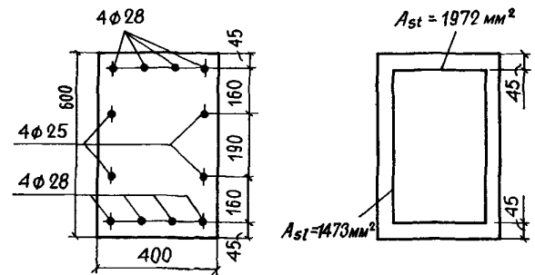
Черт. 46. К примеру расчета 28
