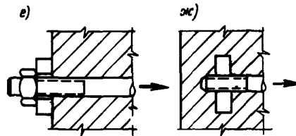
Черт. 103. Анкеровка арматуры путем устройства на концах специальных анкеров
