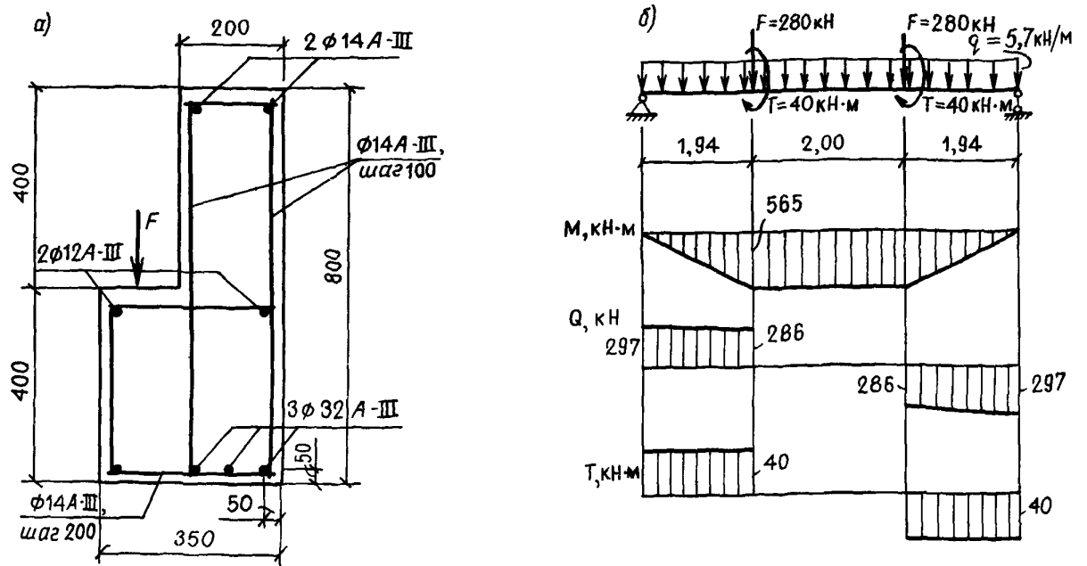
Черт. 62. К примеру расчета 47
