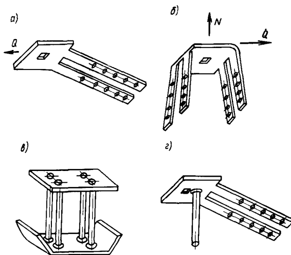
Черт. 128. Примеры конструкций закладных деталей a, б – штампованных; в, г – штампосварных
