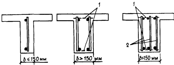
Черт. 111. Армирование балок плоскими сварными каркасами
