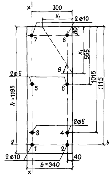
Черт. 11. К примеру расчета 12
