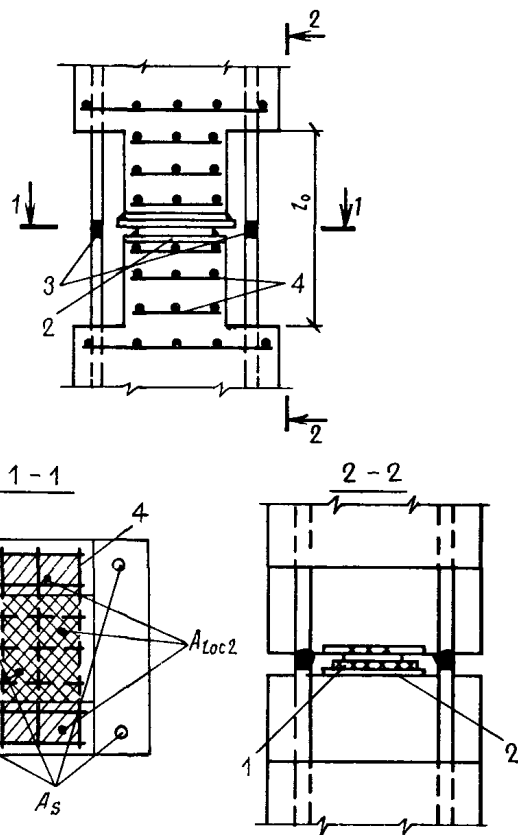
Черт. 79. Незамоноличенный стык колонны
