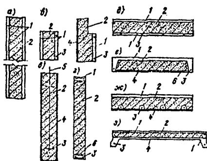
РИС. 1. ЭЛЕМЕНТЫ ИЗ АРБОЛИТА И БЕТОНА
