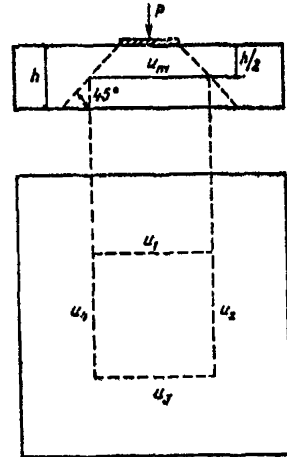
РИС. 3. СХЕМА ОБРАЗОВАНИЯ ПИРАМИДЫ ПРИ ПРОДАВЛИВАНИИ ЭЛЕМЕНТА ИЗ АРБОЛИТА
