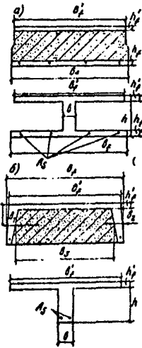
РИС. 4. СХЕМА ПОПЕРЕЧНЫХ СЕЧЕНИЙ СОСТАВНЫХ ЭЛЕМЕНТОВ
