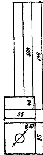
РИС. 5. СТАЛЬНАЯ БОЛВАНКА ДЛЯ ТРАПЕЗОВАНИЯ
