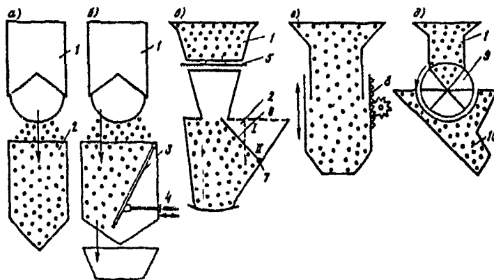
Рис. 6. СХЕМЫ ОБЪЕМНО-ВЕСОВЫХ ДОЗАТОРОВ (по данным ВНИИЖелезобетон)
