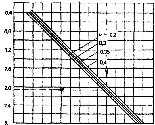
Номограмма для определения значений \delta_0
