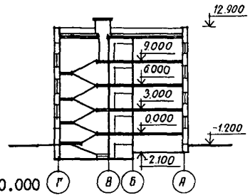
РАЗРЕЗ I-I
