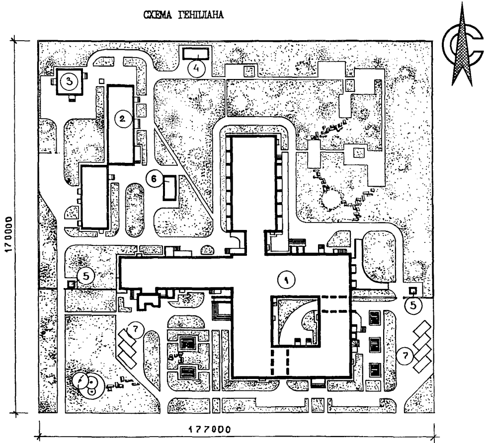
ЭКСПЛИКАЦИЯ ЗДАНИЙ И СООРУЖЕНИЙ
