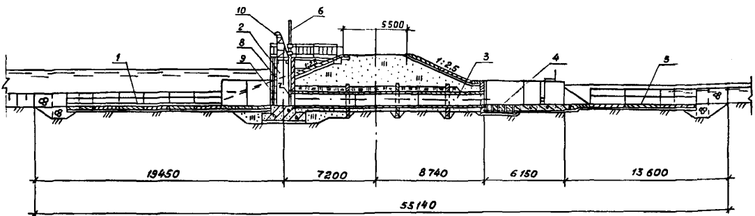
РАЗРЕЗ I-I
