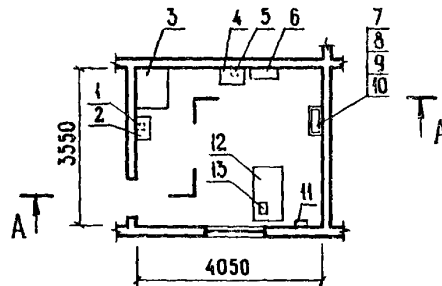
ПЛАН НА ОТМ.0.00 С РАЗМЕЩЕНИЕМ ОБОРУДОВАНИЯ
