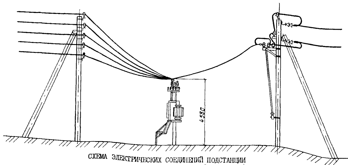
ПРИСОЕДИНЕНИЕ ВЛ 10 и 0,4 кВ К ПОДСТАНЦИИ С ВОЗДУШНЫМИ ВВОДАМИ
