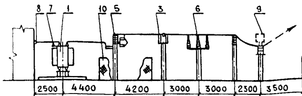
РАЗРЕЗ I-I
