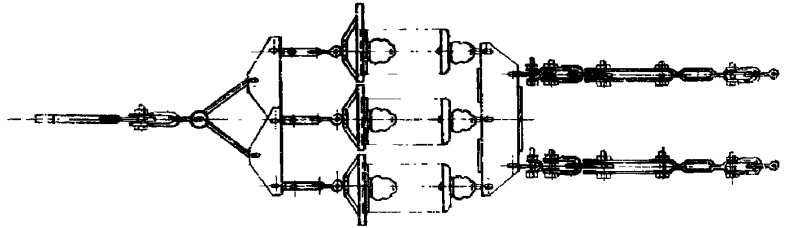
ГИРЛЯНДЫ НАТЯЖНЫЕ
