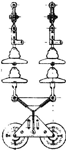
ГИРЛЯНДЫ ПОДДЕРЖИВАЮЩИЕ
